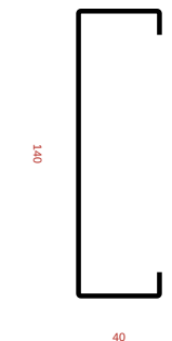
Ue 140x40x12x0,80
