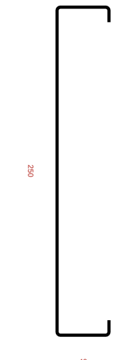
Ue 250x40x12x1,25
