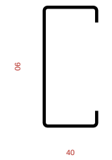
Ue 90x40x12x1,25
