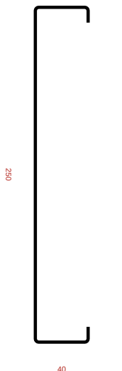
Ue 250x40x12x1,25
