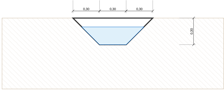
vala 300 x 300, fundo 1:1, 1% — 200 3 L/s (projeto 1:3 1 L/s), todo no fundo para a água correr
