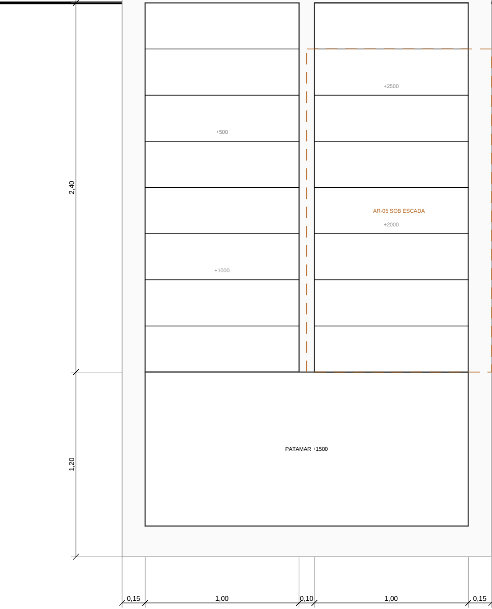
1 PLANTA DA ESCADA ESCALA 1:25
