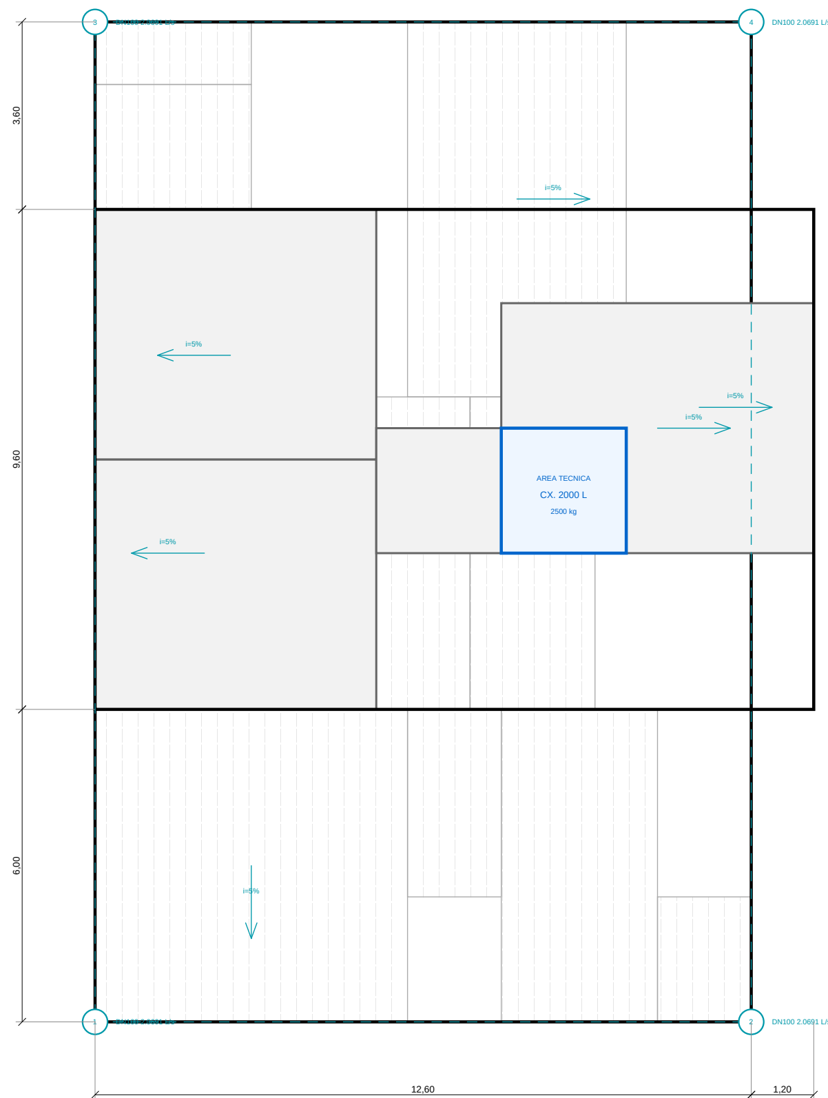
1 COBERTURA ESCALA 1:100
