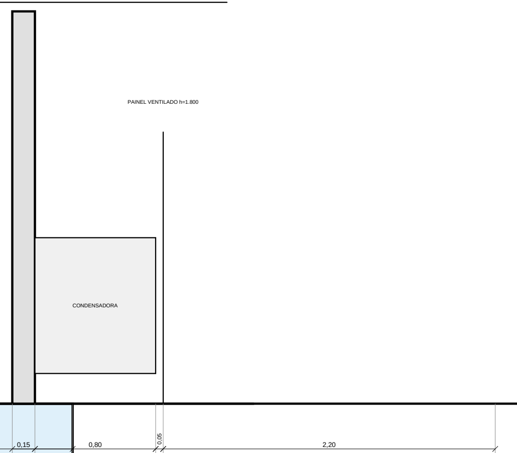
4 FAIXA TECNICA LATERAL — CORTE ESCALA 1:25
