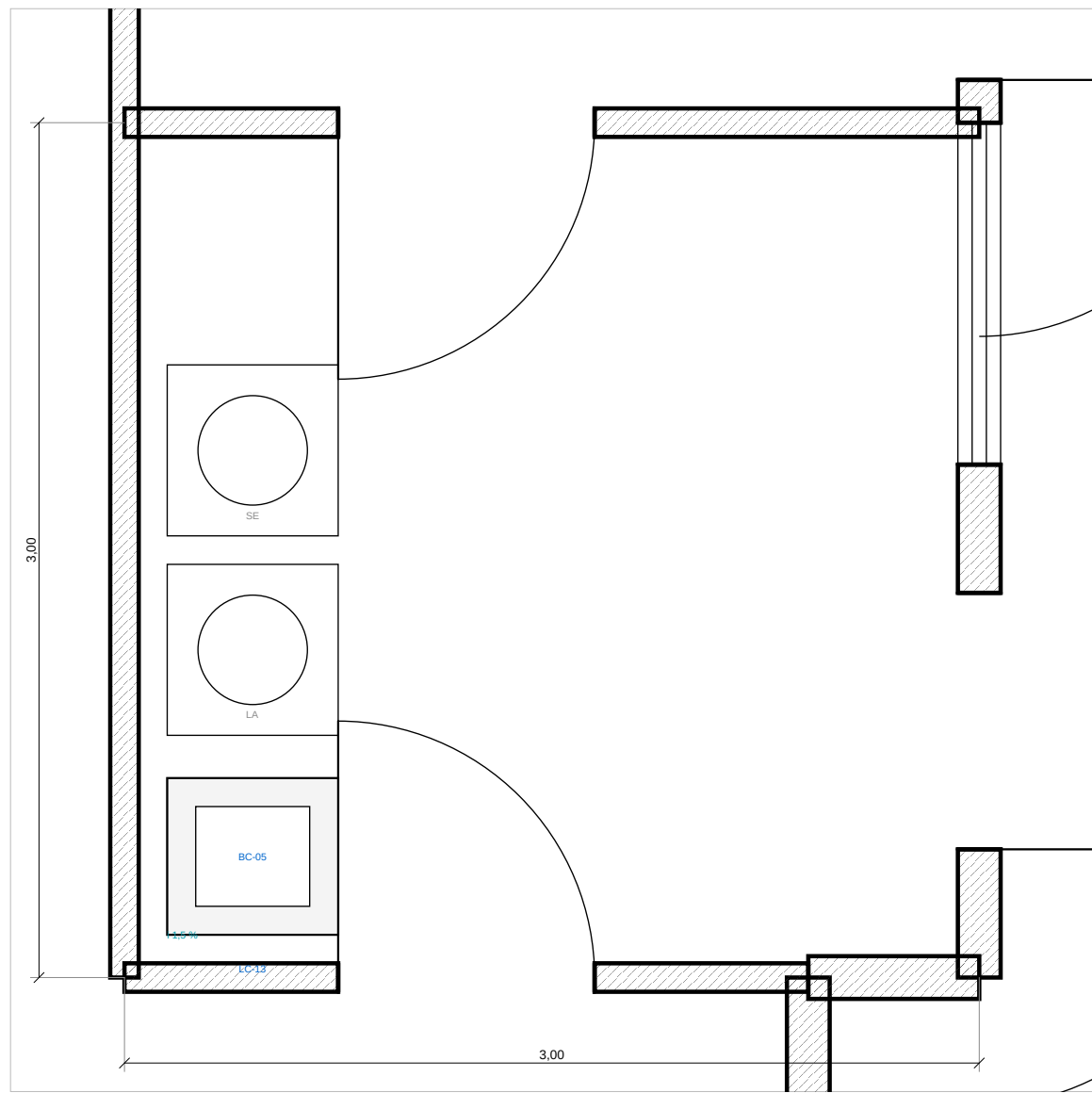
2 LAVANDERIA ESCALA 1:25
