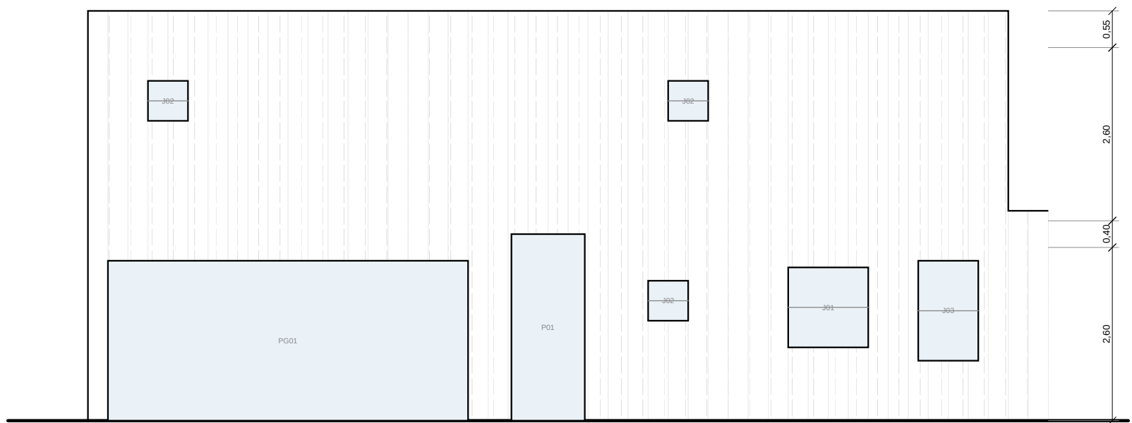
FACHADA FRONTAL (SUL)
