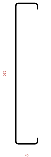
Ue 250x40x12x2,25
