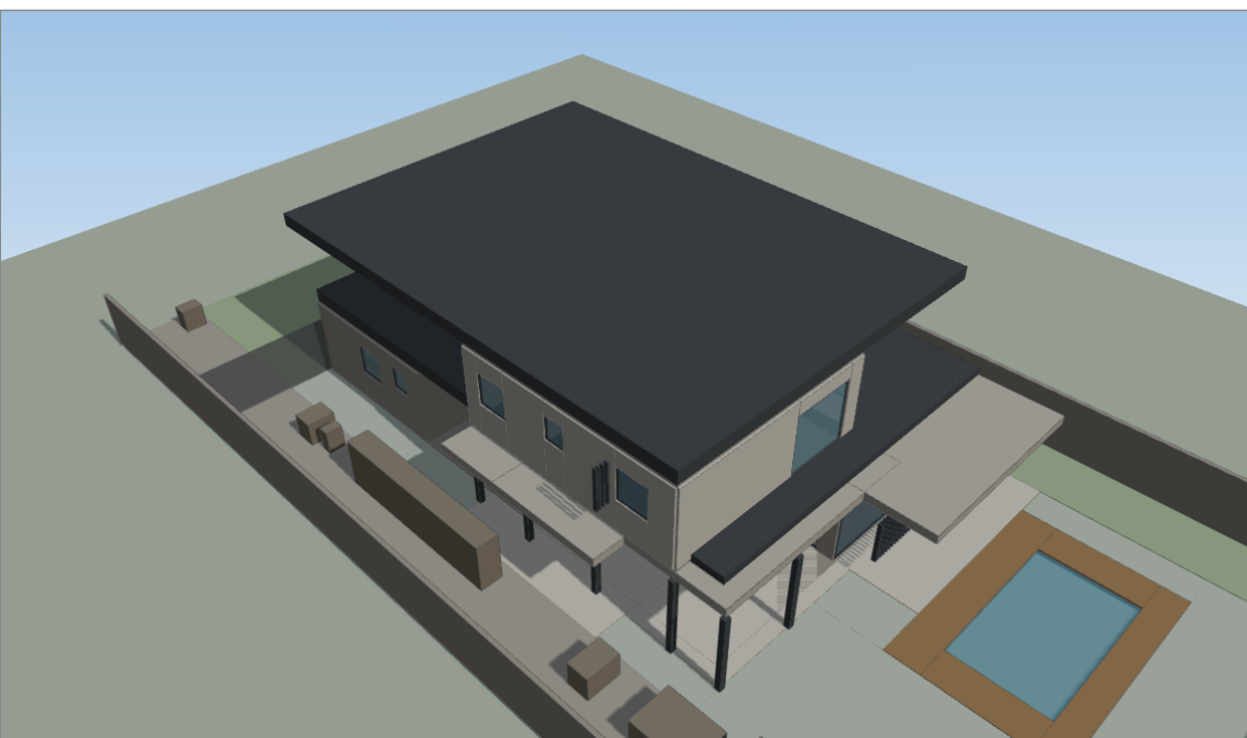
13. VISTA AÉREA DO NOROESTE — Azimute: 315° (0.00°) — Tax 30° Câmera (43.0, 38.0, +4.500 m)
