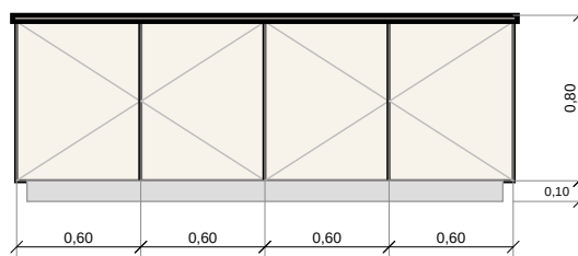
5 BC-06 GABINETE SOB GRANITO ESCALA 1:40
