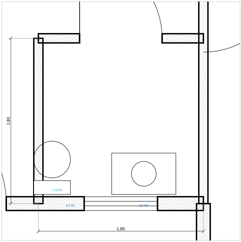
1 BANHO SOCIAL ESCALA 1:25
