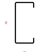
Ue 90x40x12x1,25
