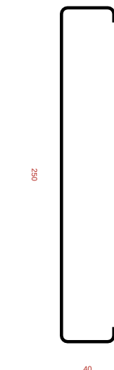
Ue 250x40x12x2,25
