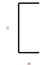
U 92x38x0,95
