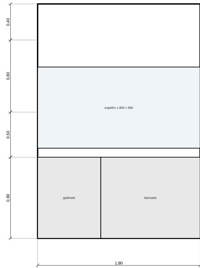
LAVABO SOCIAL — PAREDE DA BANCADA
