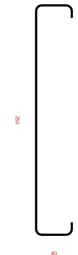
Ue 250x40x15x3,00
