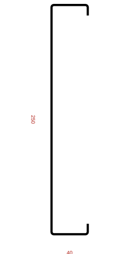
Ue 250x40x12x1,25
