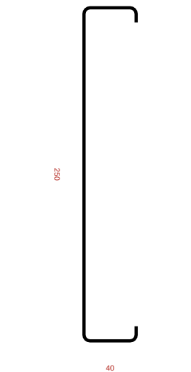
Ue 250x40x12x2,25
