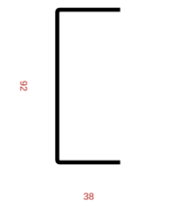
U 92x38x0,95
