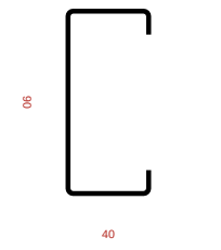
Ue 90x40x12x1,25
