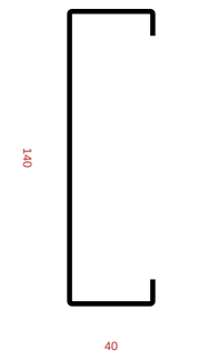
Ue 140x40x12x0,80
