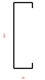
Ue 140x40x12x0,80
