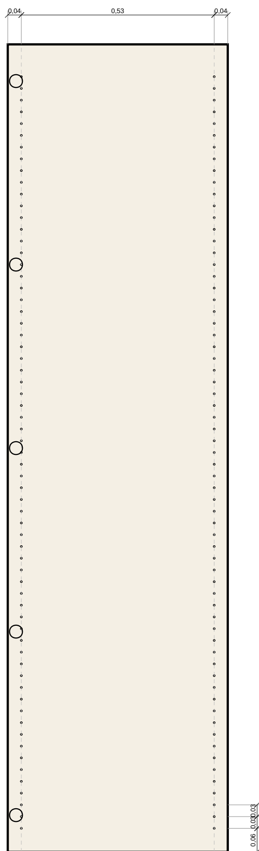
A LATERAL TIPICA 600 x 2.200 — FURCAO SISTEMA 32 E CANECOS ESCALA 1:10
