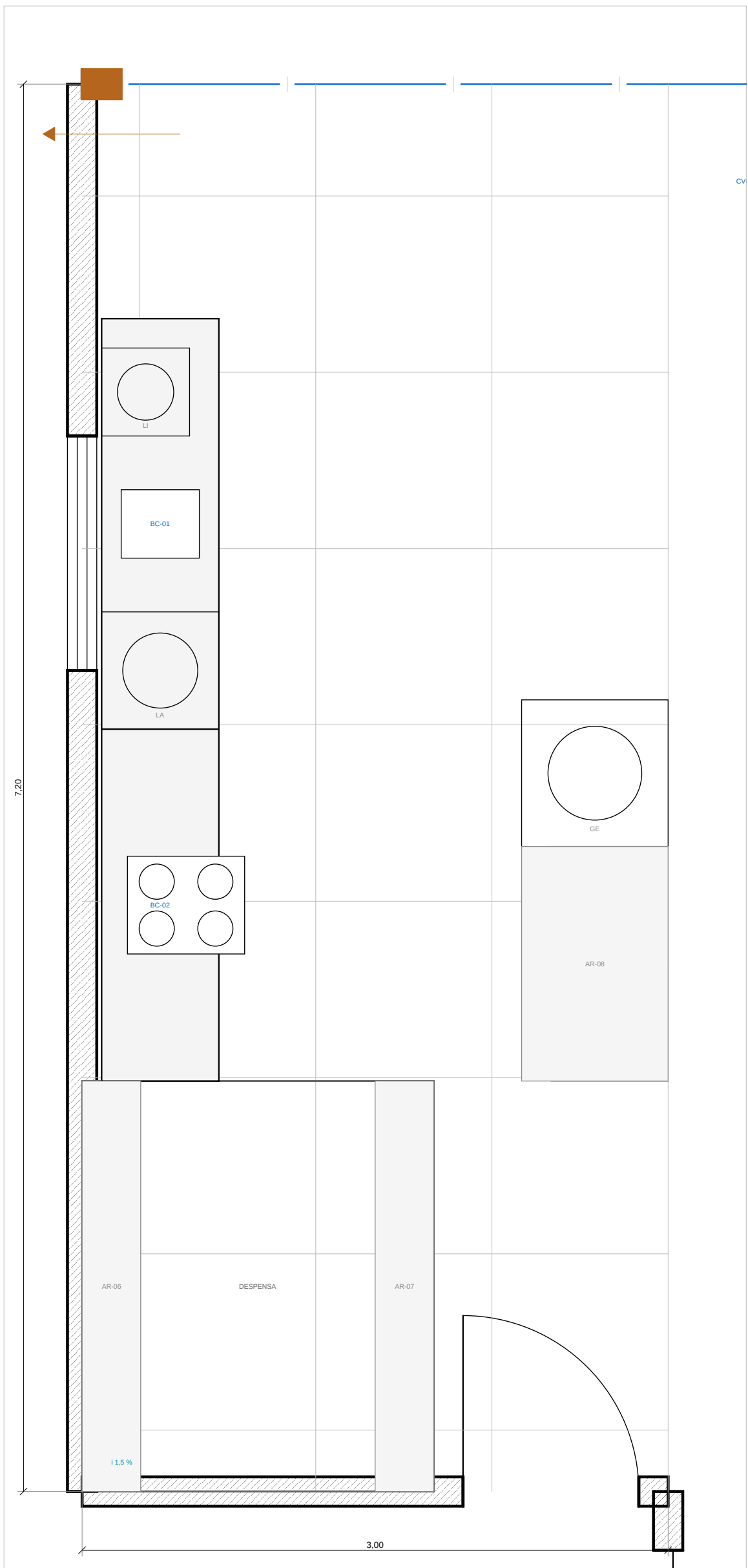
3 COZINHA ESCALA 1:25
