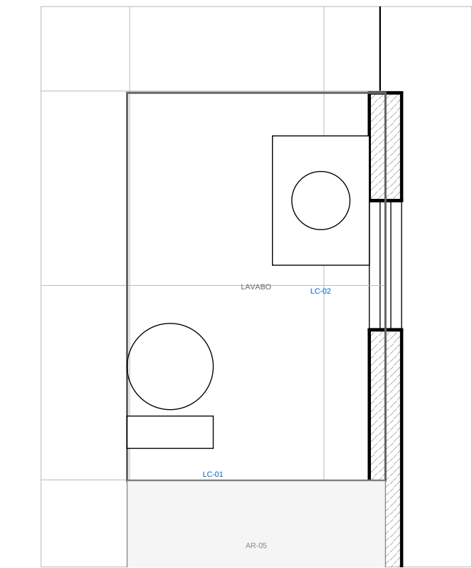
1 LAVABO SOB A ESCADA ESCALA 1:25
