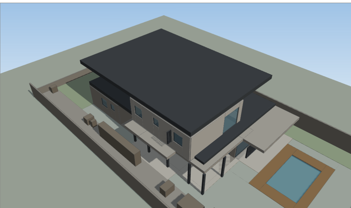
13. VISTA AEREA DO NOROESTE 1 - AZIMUTH - 001.000 - 001.500° CAMERA (20.0, 20.0, 14.000 m)
