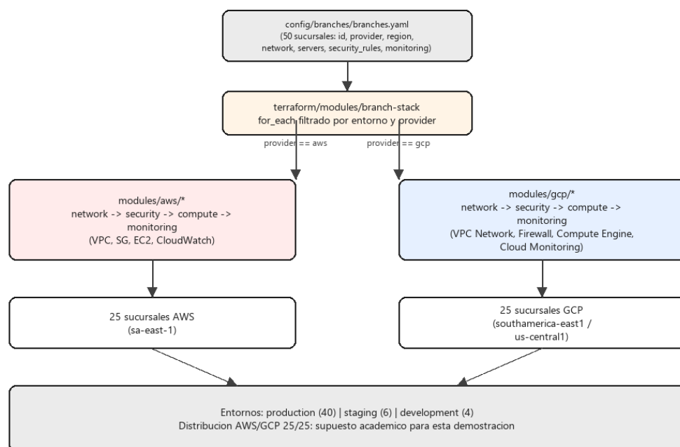
Figura 1. Arquitectura general - 50 sucursales multi-cloud
