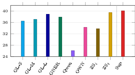
AMI ( \uparrow )
