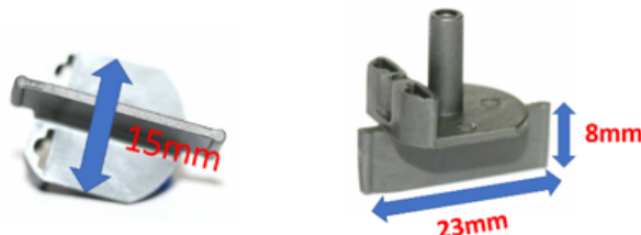
FIGURE 7 – Dimensions du guide
