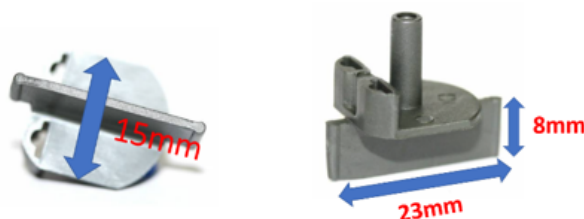
FIGURE 3 – Dimensions du guide
