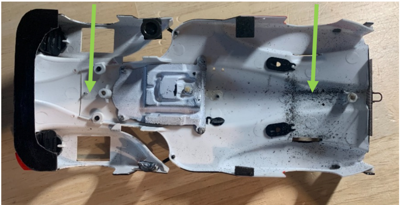
FIGURE 4 – Position des poids additionnels
