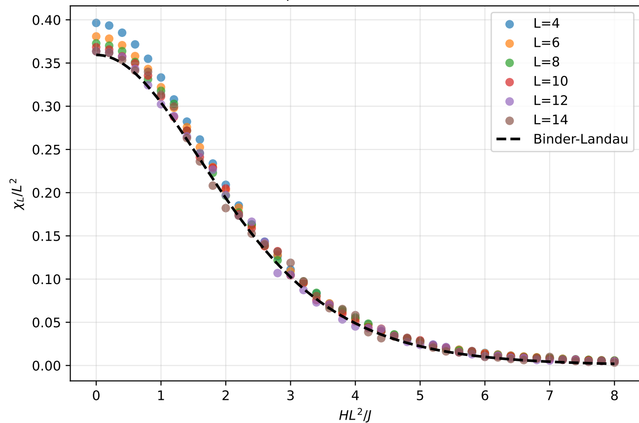
Susceptibilité réduite, T = 2.1
