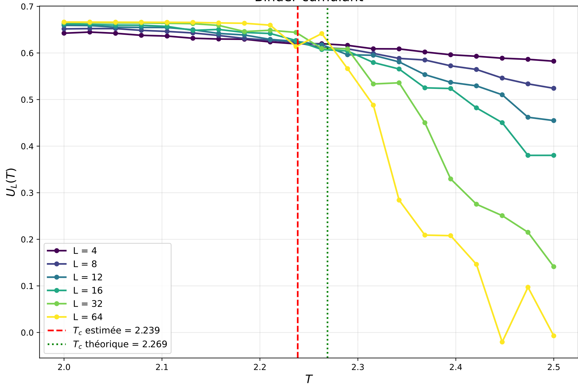
Binder cumulant
