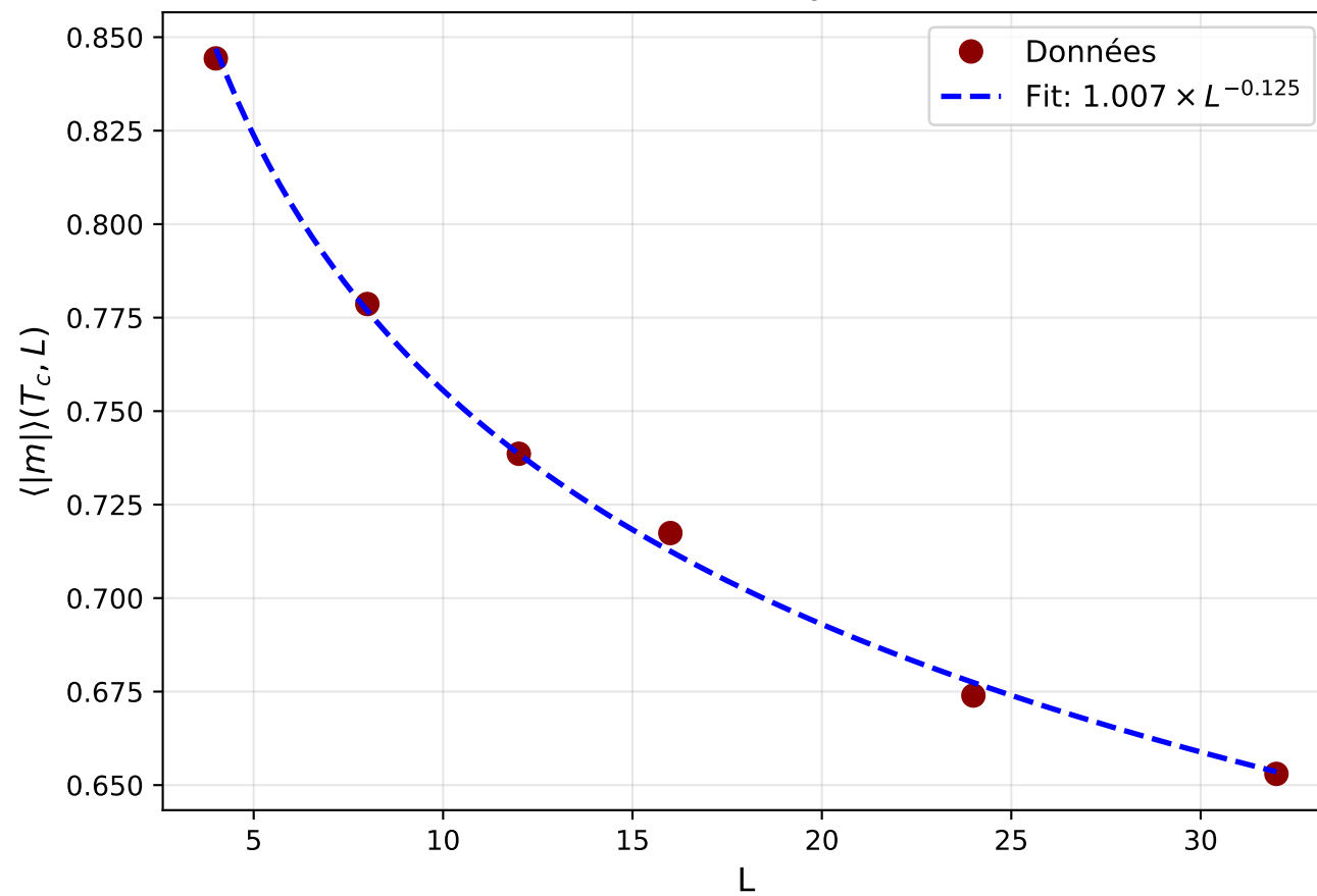
Aimantation à T_c = 2.269
