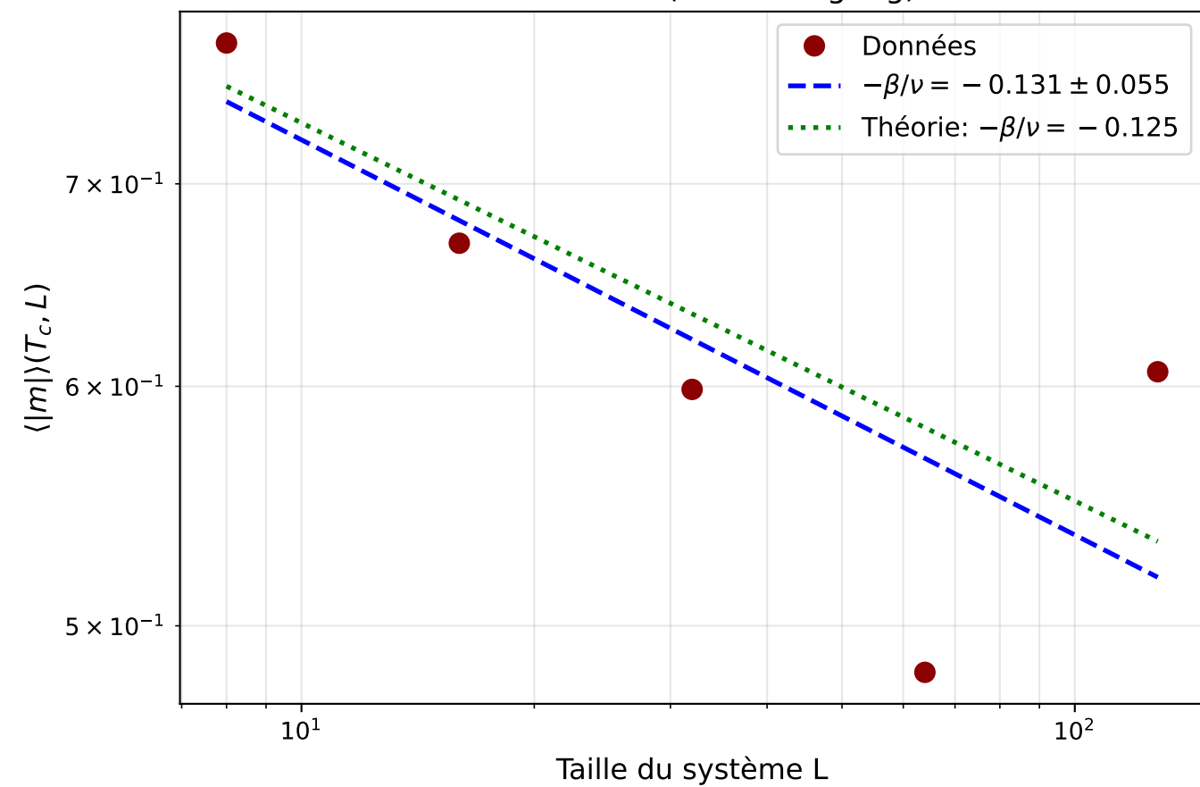
Aimantation (échelle log-log)
