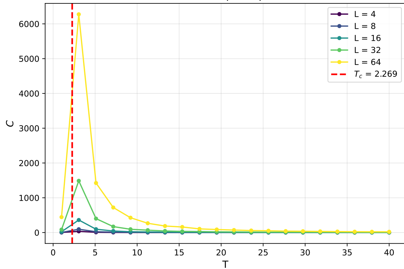
Chaleur spécifique
