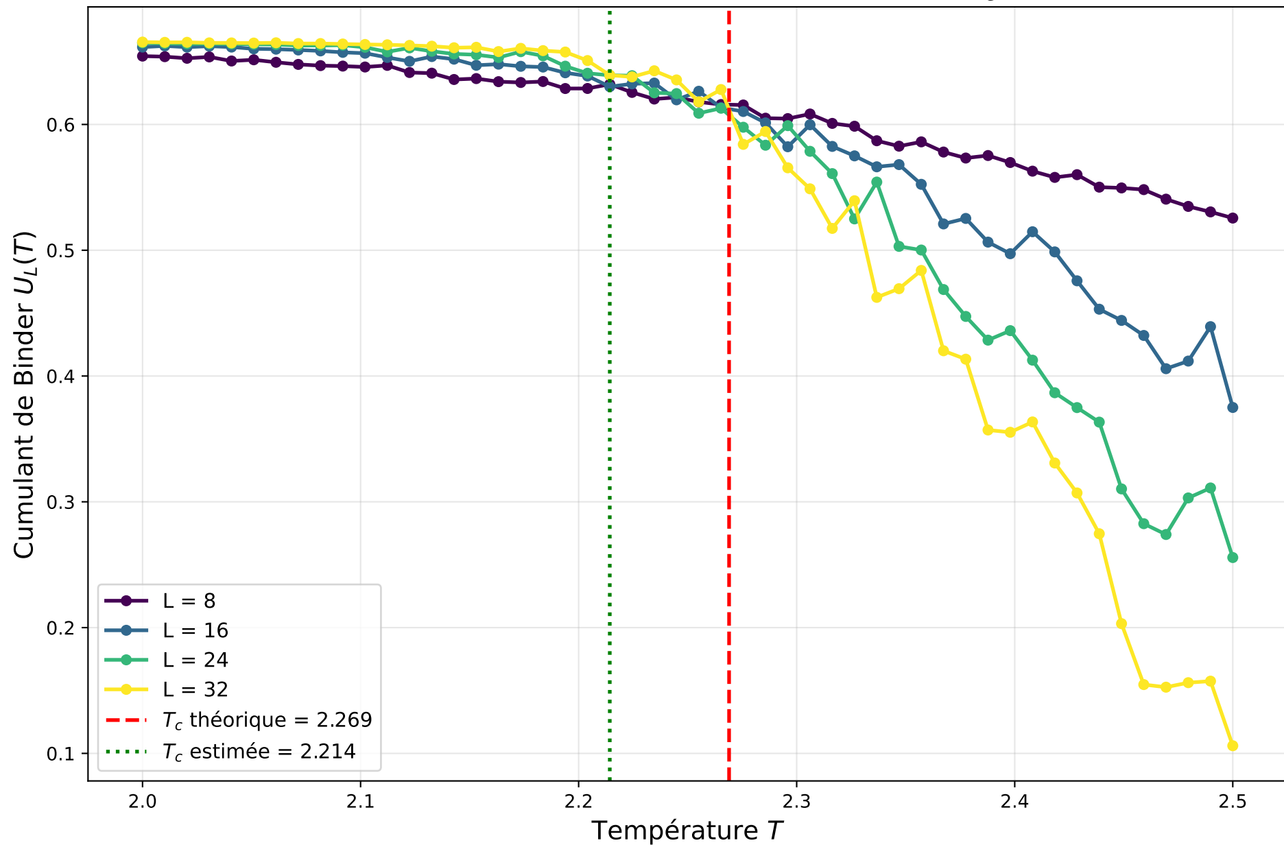
Cumulant de Binder - Détermination de T_c
