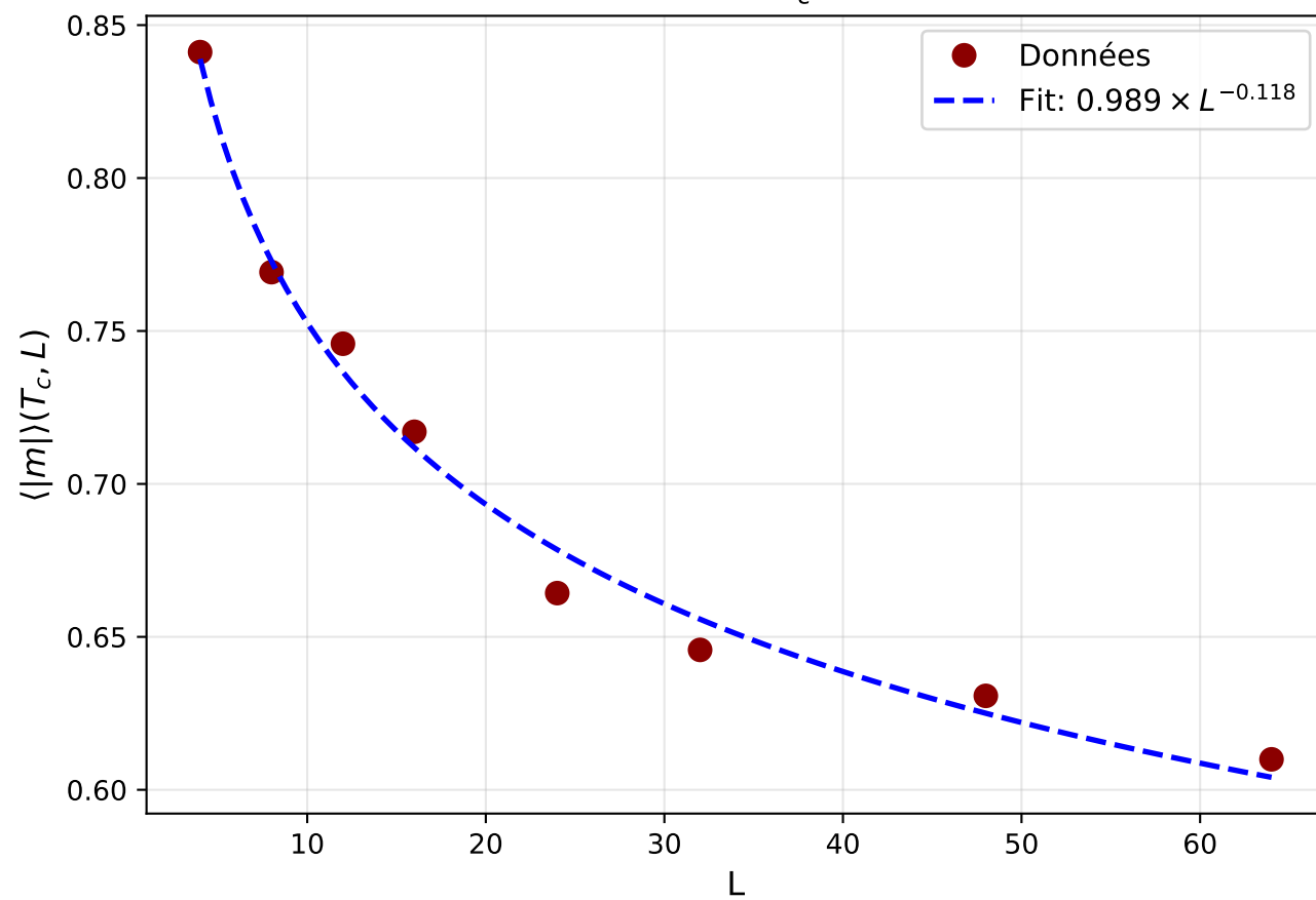
Aimantation à T_c = 2.269
