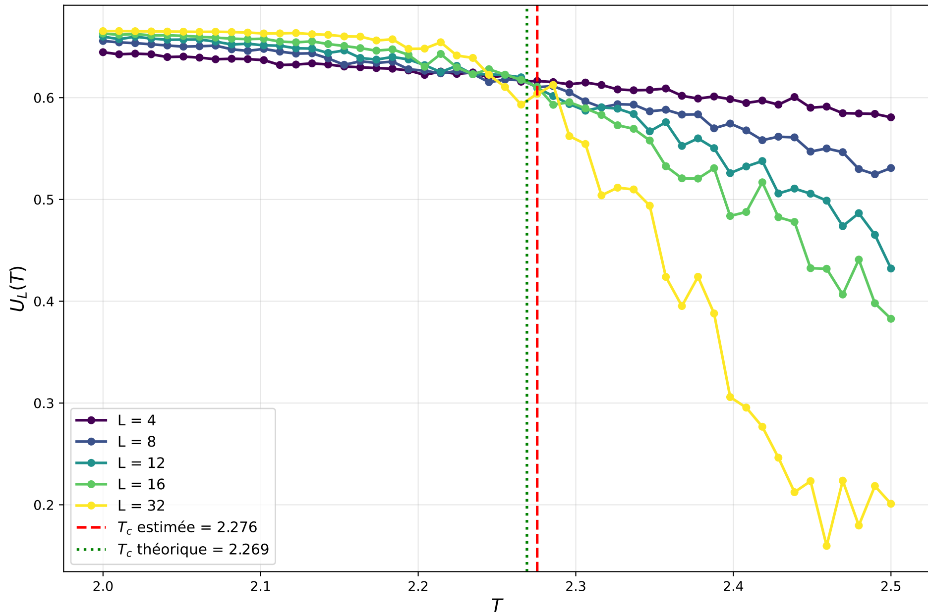
Binder cumulant
