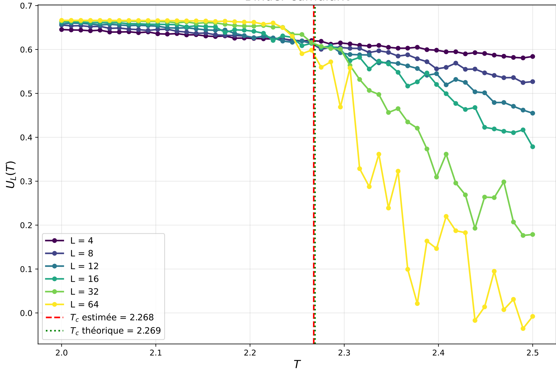
Binder cumulant
