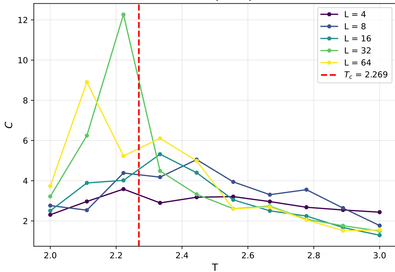
Chaleur spécifique
