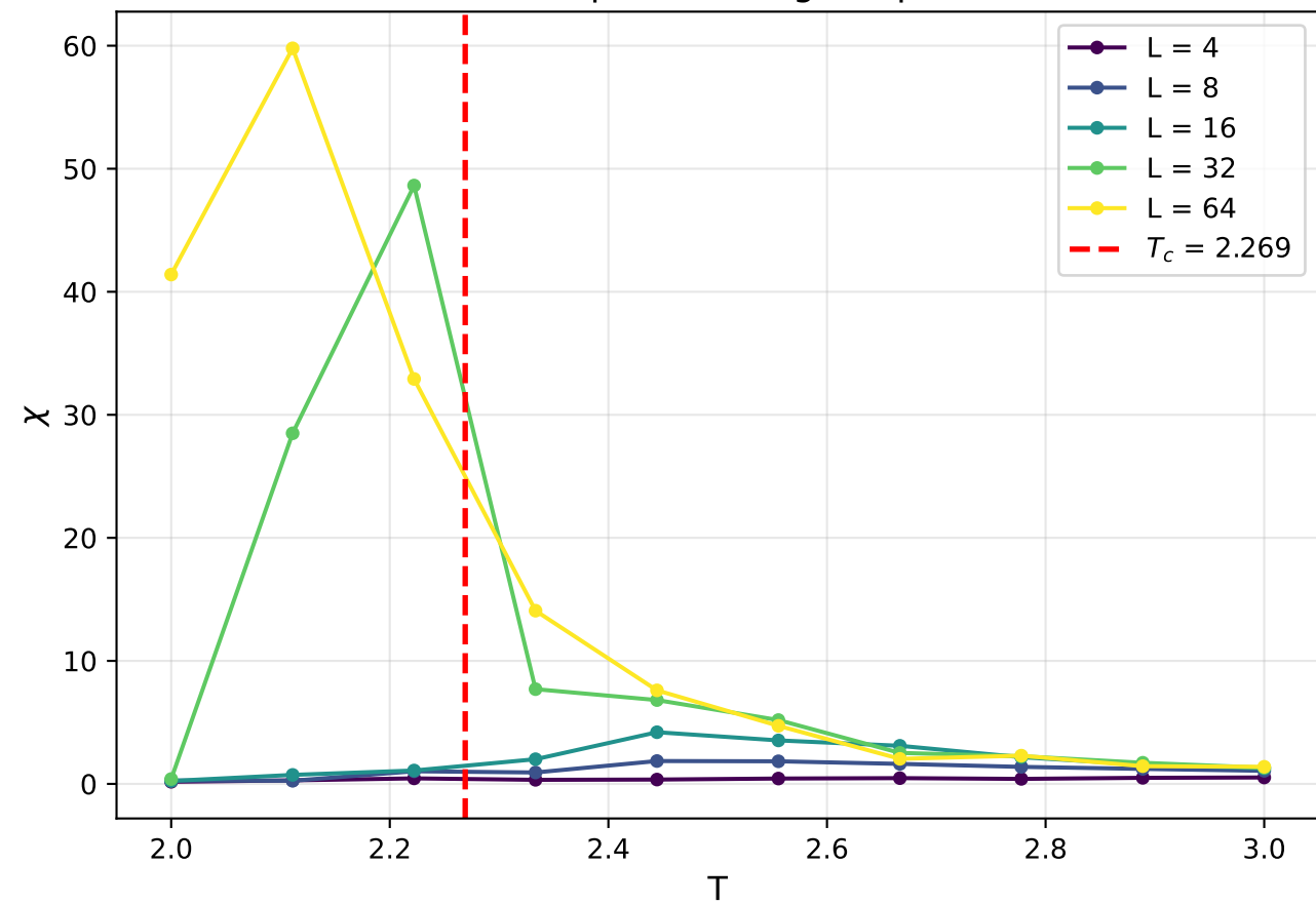
Susceptibilité magnétique
