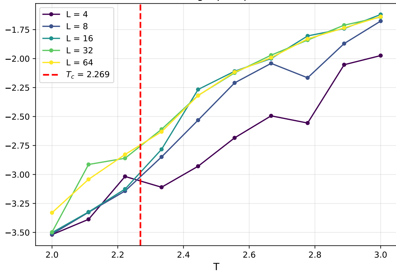
Chaleur spécifique
