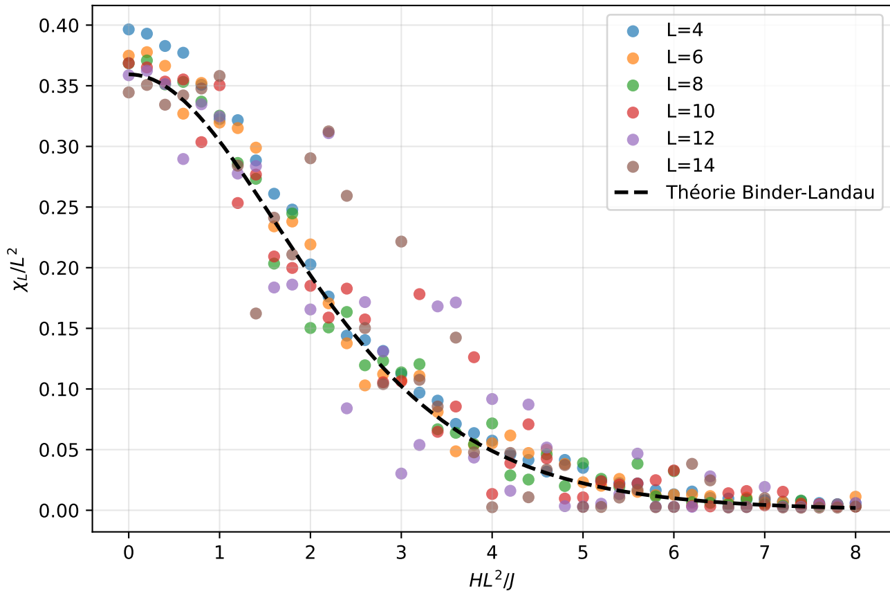
Susceptibilité scalée, T = 2.1
