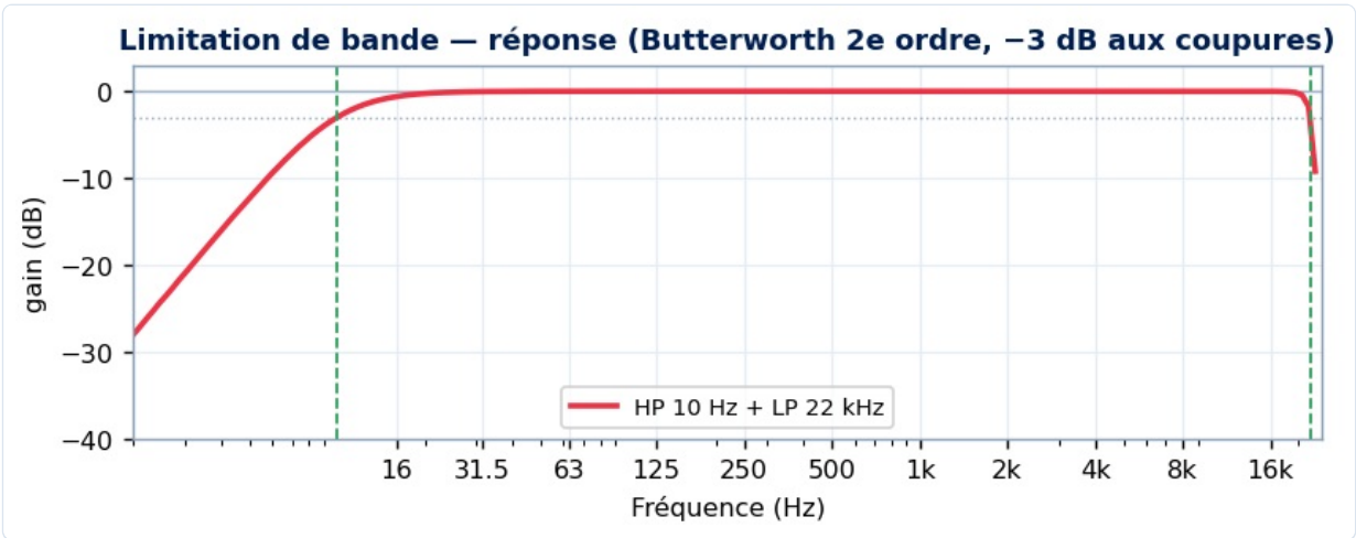
Limitation de bande — réponse ( -3\text{ dB} aux coupures).
