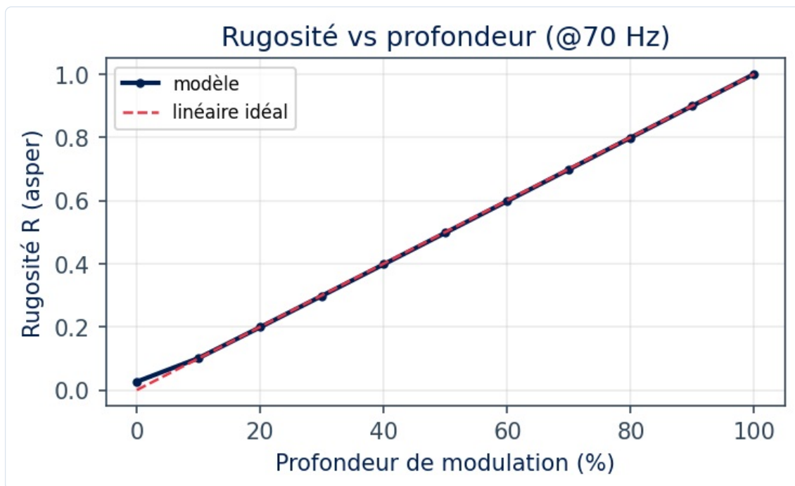
Rugosité vs profondeur de modulation (@70 Hz) — réponse linéaire.
