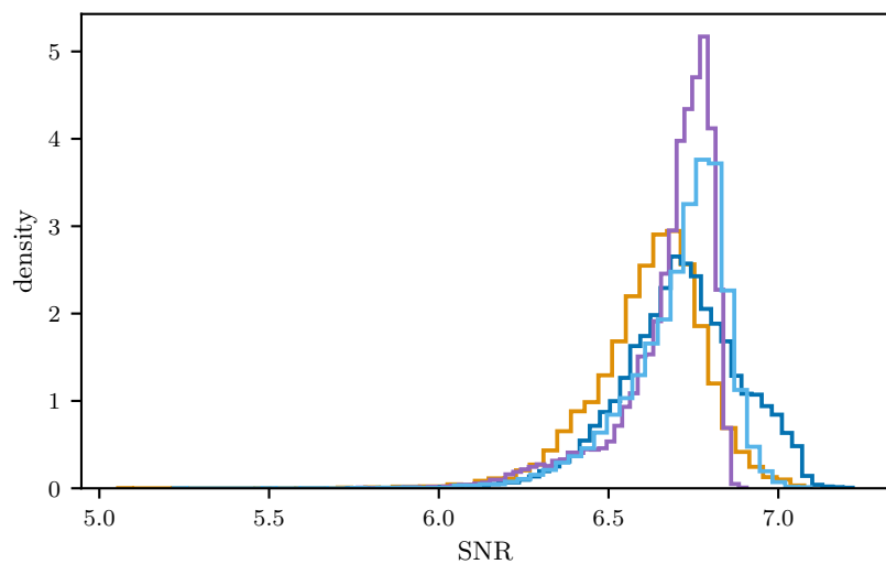
network SNR (optimal, \sqrt{H^2 + L^2} )
