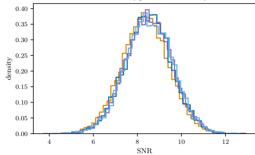
network SNR (optimal, \sqrt{H^2 + L^2} )
