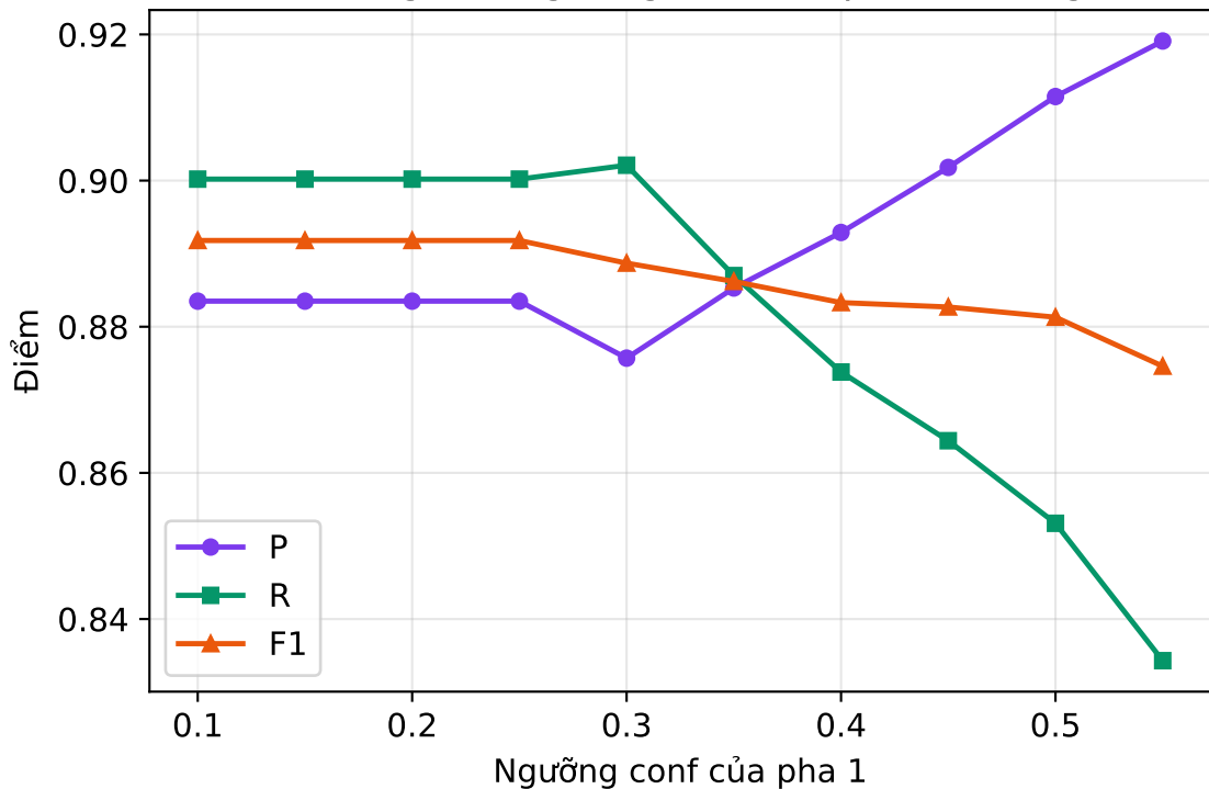
Ảnh hưởng của ngưỡng conf lên phát hiện người
