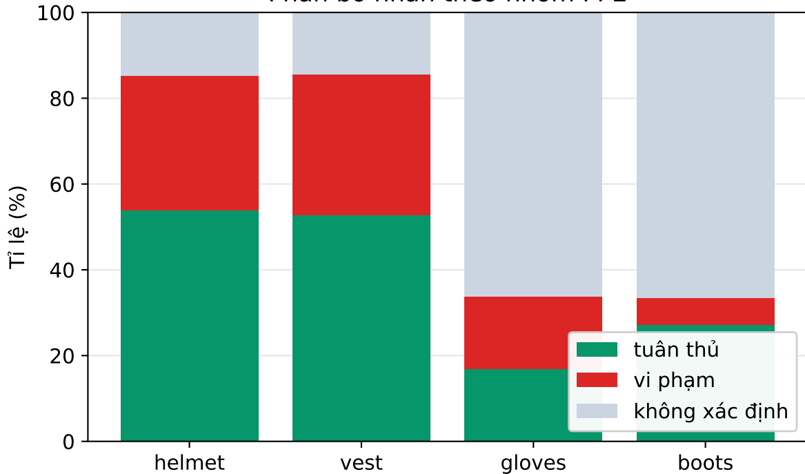
Phân bố nhân theo nhóm PPE
