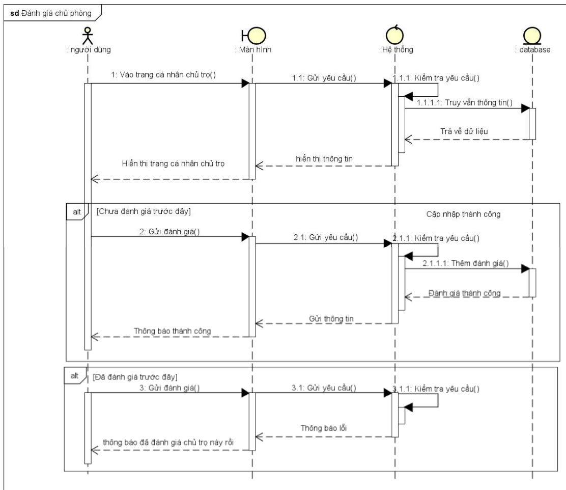
Hình 3.2-27. Hình sơ đồ tuần tự chức năng đánh giá
