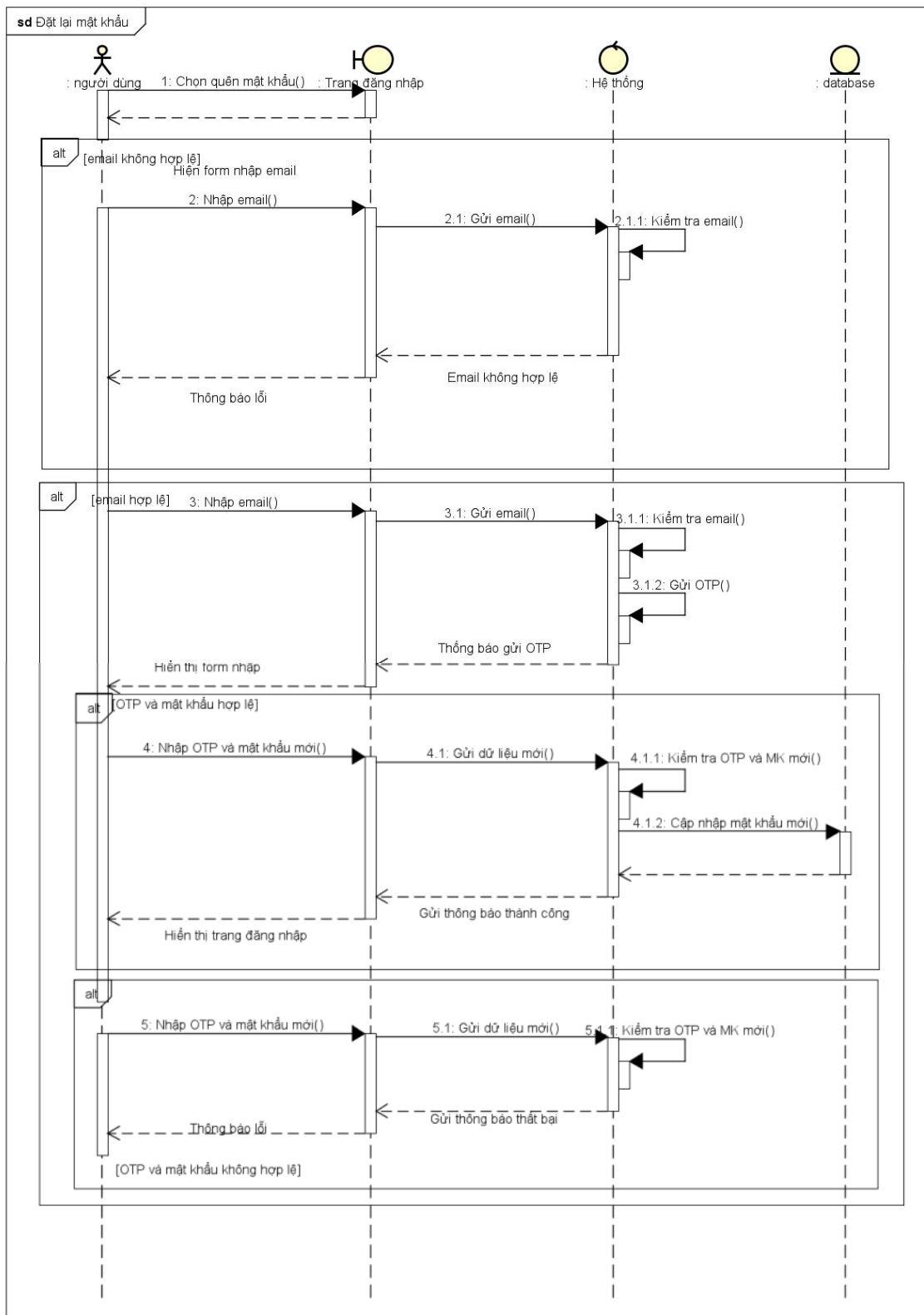
Hình 3.2-18. Hình sơ đồ tuần tự chức năng đặt lại mật khẩu
