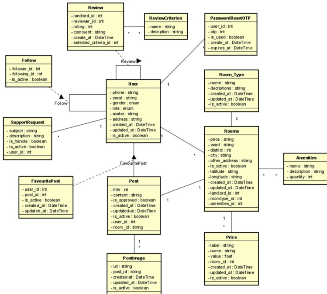
Hình 3.2-1. Sơ đồ lớp
