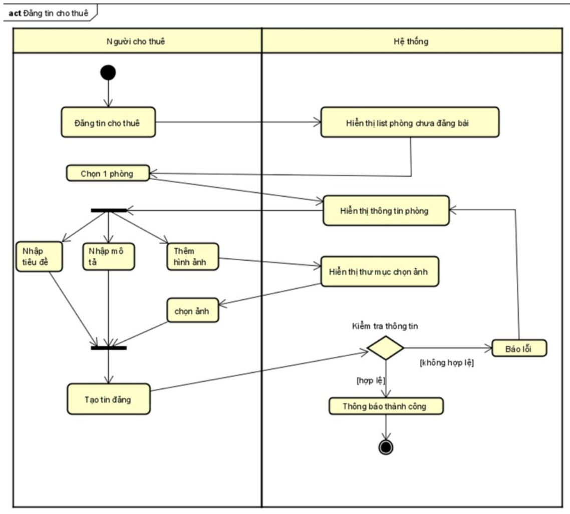
Hình 3.2-8. Sơ đồ activity chức năng đăng tin
