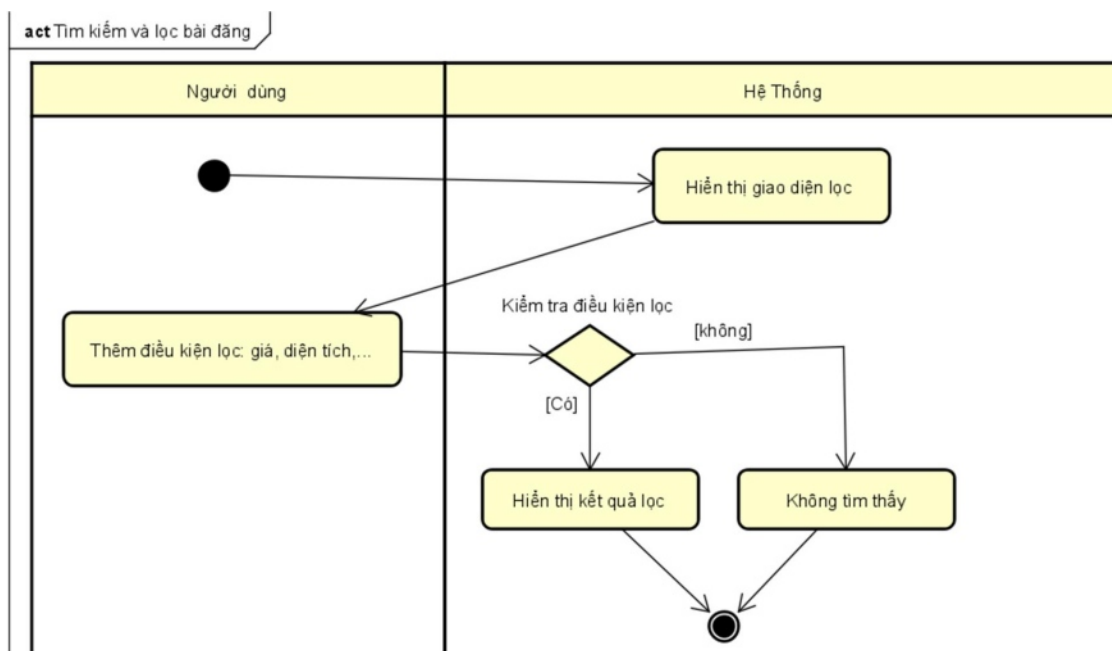
Hình 3.2-5. Sơ đồ activity chức năng tìm kiếm và lọc
