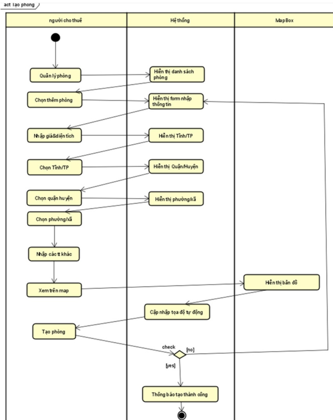
Hình 3.2-13. Sơ đồ activity chức năng thêm phòng
