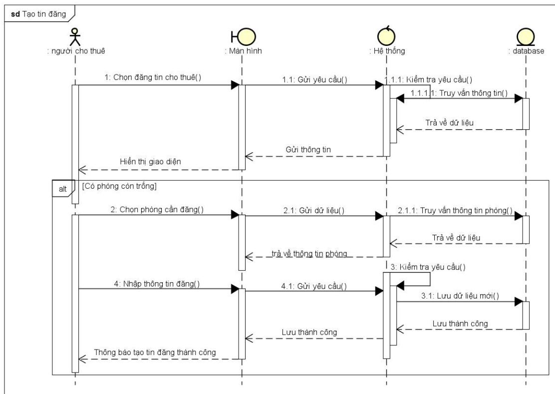
Hình 3.2-23. Hình sơ đồ tuần tự chức năng tạo tin đăng
