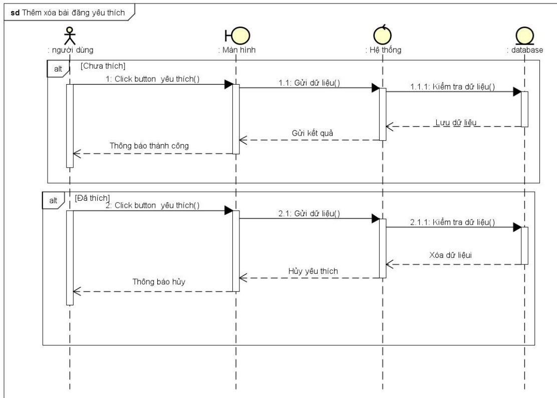
Hình 3.2-22. Hình sơ đồ tuần tự chức năng thêm, xóa bài đăng yêu thích
