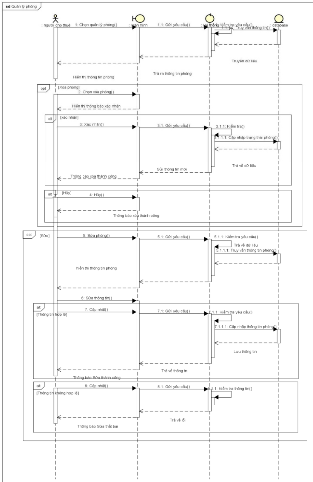
Hình 3.2-21. Hình sơ đồ tuần tự chức năng quản lý phòng
