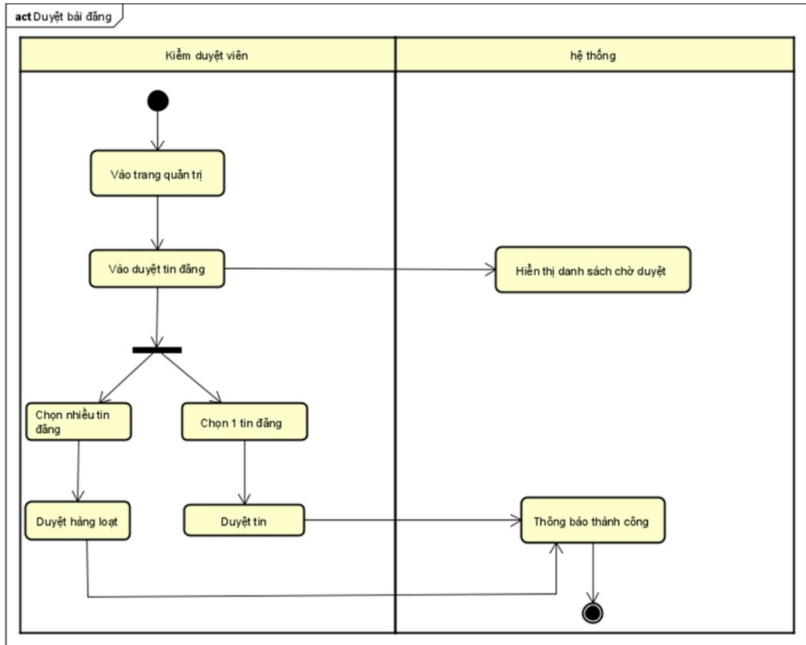
Hình 3.2-9. Sơ đồ activity chức năng duyệt tin đăng
