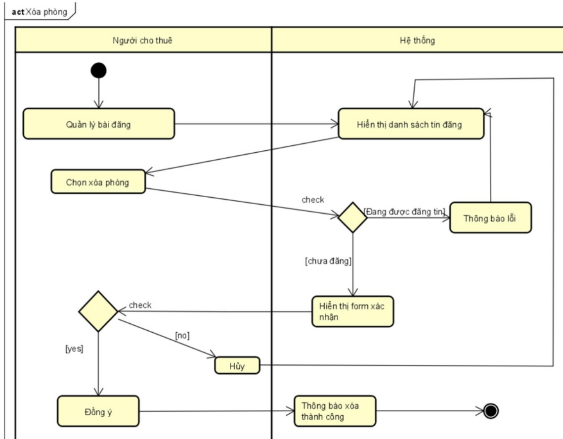
Hình 3.2-14. Sơ đồ activity chức năng xóa phòng
