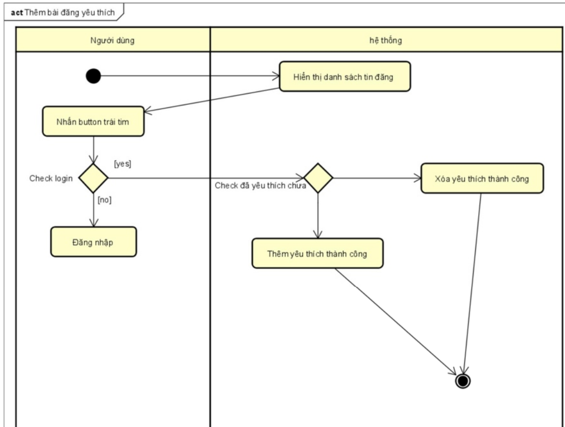
Hình 3.2-12. Sơ đồ activity chức năng thêm bài đ ăng yêu thích
