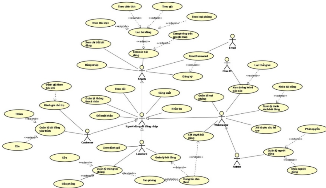
Hình 3.2-2. Sơ đồ use case tổng quát
