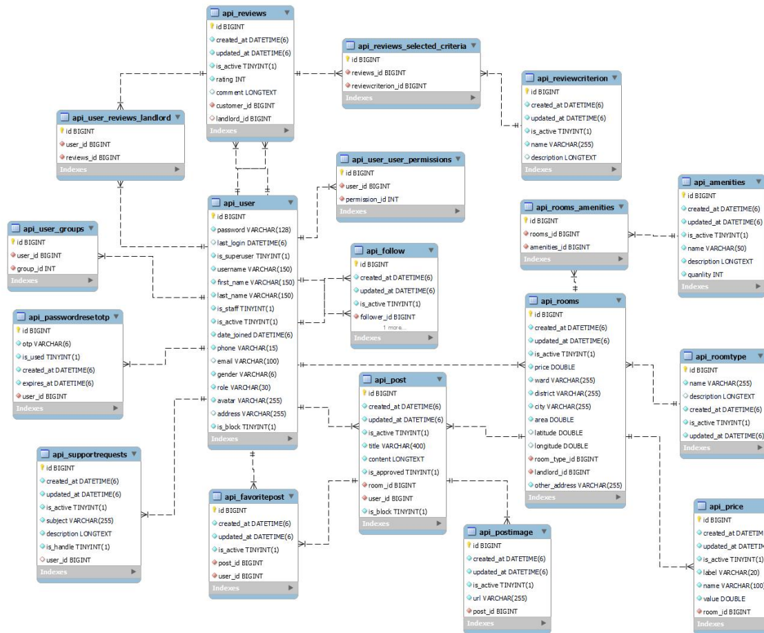
Hình 3.2-15. Lược đồ cơ sở dữ liệu
