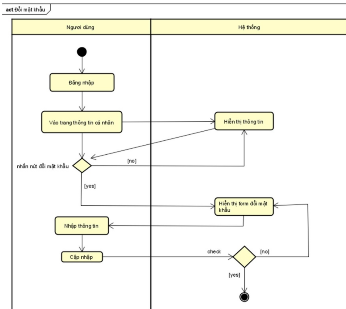
Hình 3.2-7. Sơ đồ activity chức năng đổi mật khẩu
