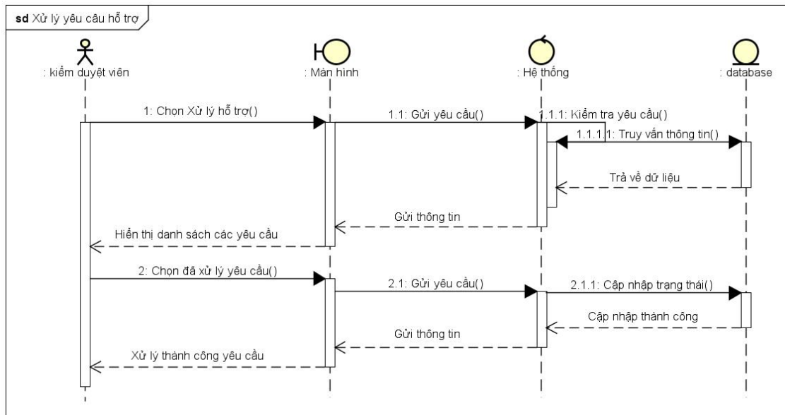
Hình 3.2-29. Hình sơ đồ tuần tự xử lý yêu cầu hỗ trợ
