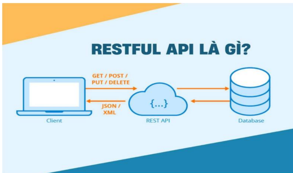
Hình 2.3-1. Hình kiến trúc RESTful API (Nguồn: Trích dẫn[8])
