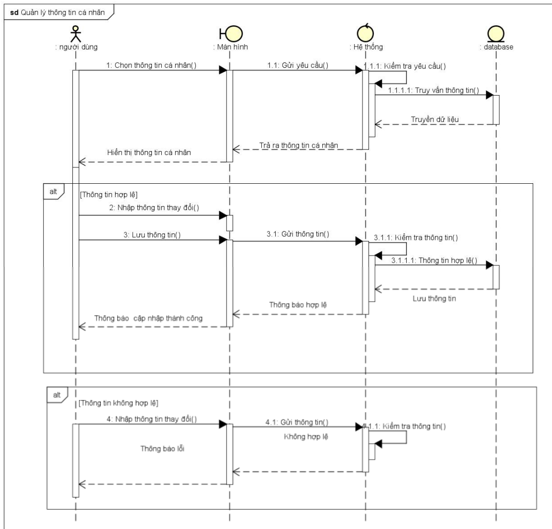
Hình 3.2-20. Hình sơ đồ tuần tự chức năng quản lý thông tin cá nhân
