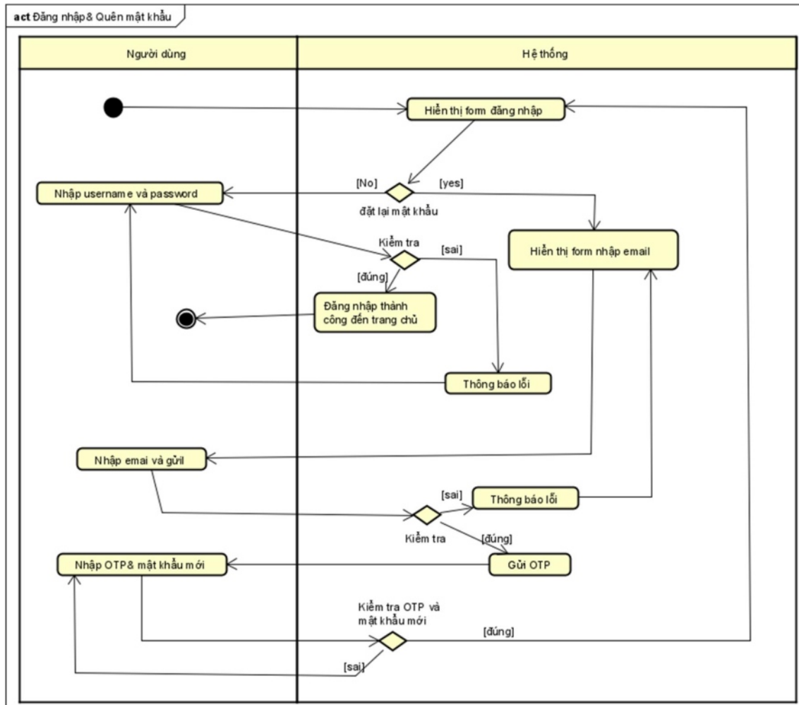
Hình 3.2-3. Sơ đồ activity đăng nhập và đặt lại mật khẩu
