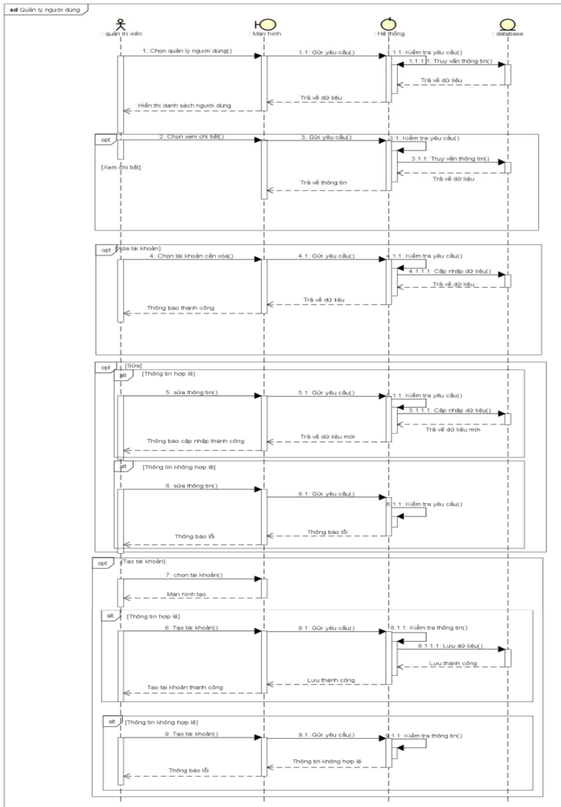
Hình 3.2-28. Hình sơ đồ tuần tự chức năng quản lý người dùng
