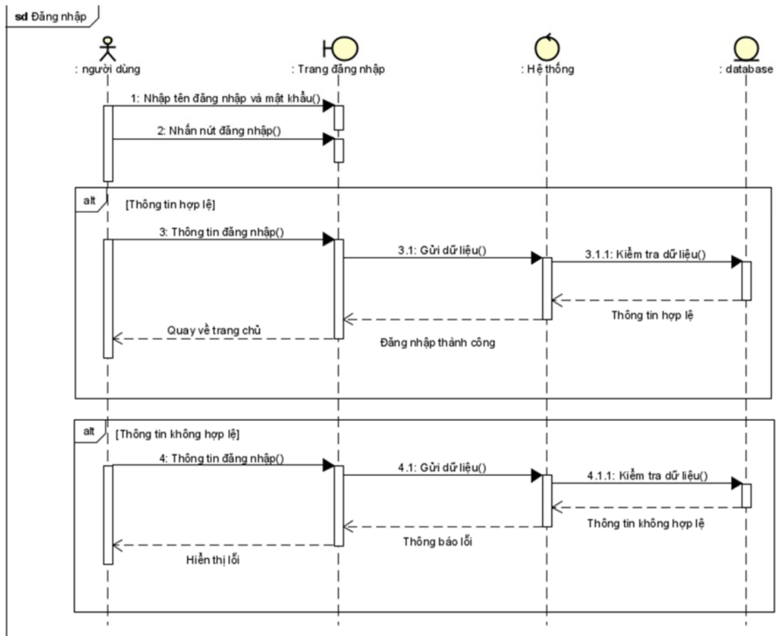
Hình 3.2-16. Hình sơ đồ tuần tự chức năng đăng nhập
