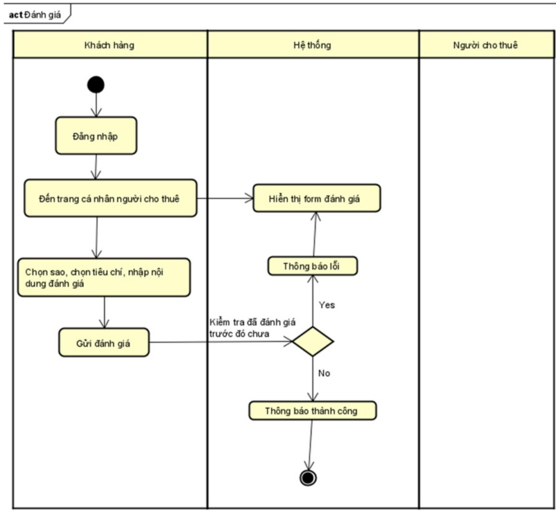
Hình 3.2-10. Sơ đồ activity chức năng đánh giá
