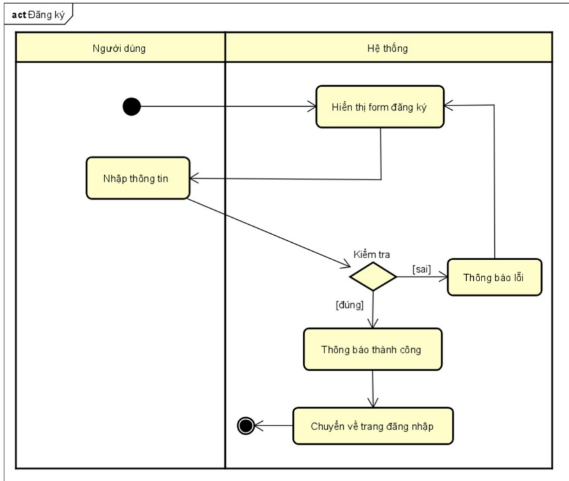
Hình 3.2-4. Sơ đồ activity chức năng đăng ký
