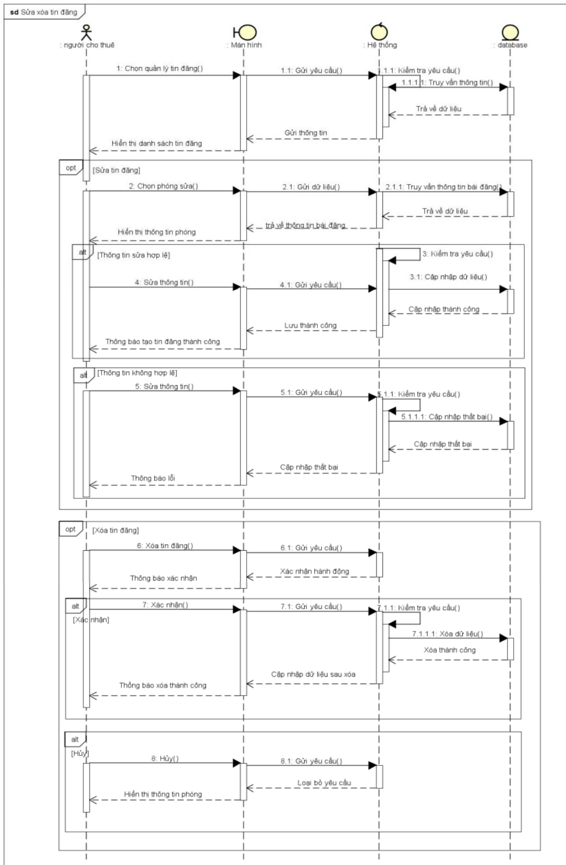
Hình 3.2-24. Hình sơ đồ tuần tự chức năng sửa, xóa tin đăng
