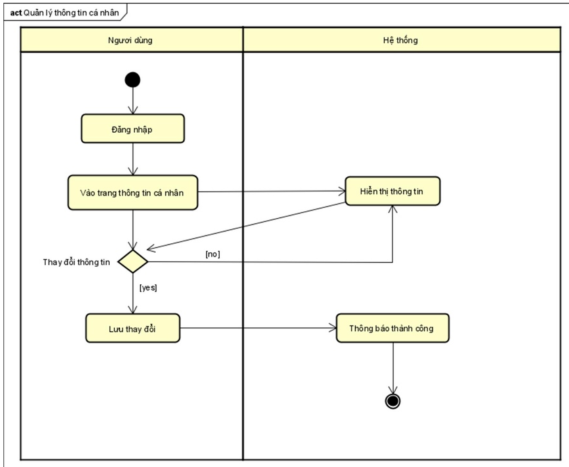
Hình 3.2-11. Sơ đồ activity chức năng quản lý thông tin cá nhân
