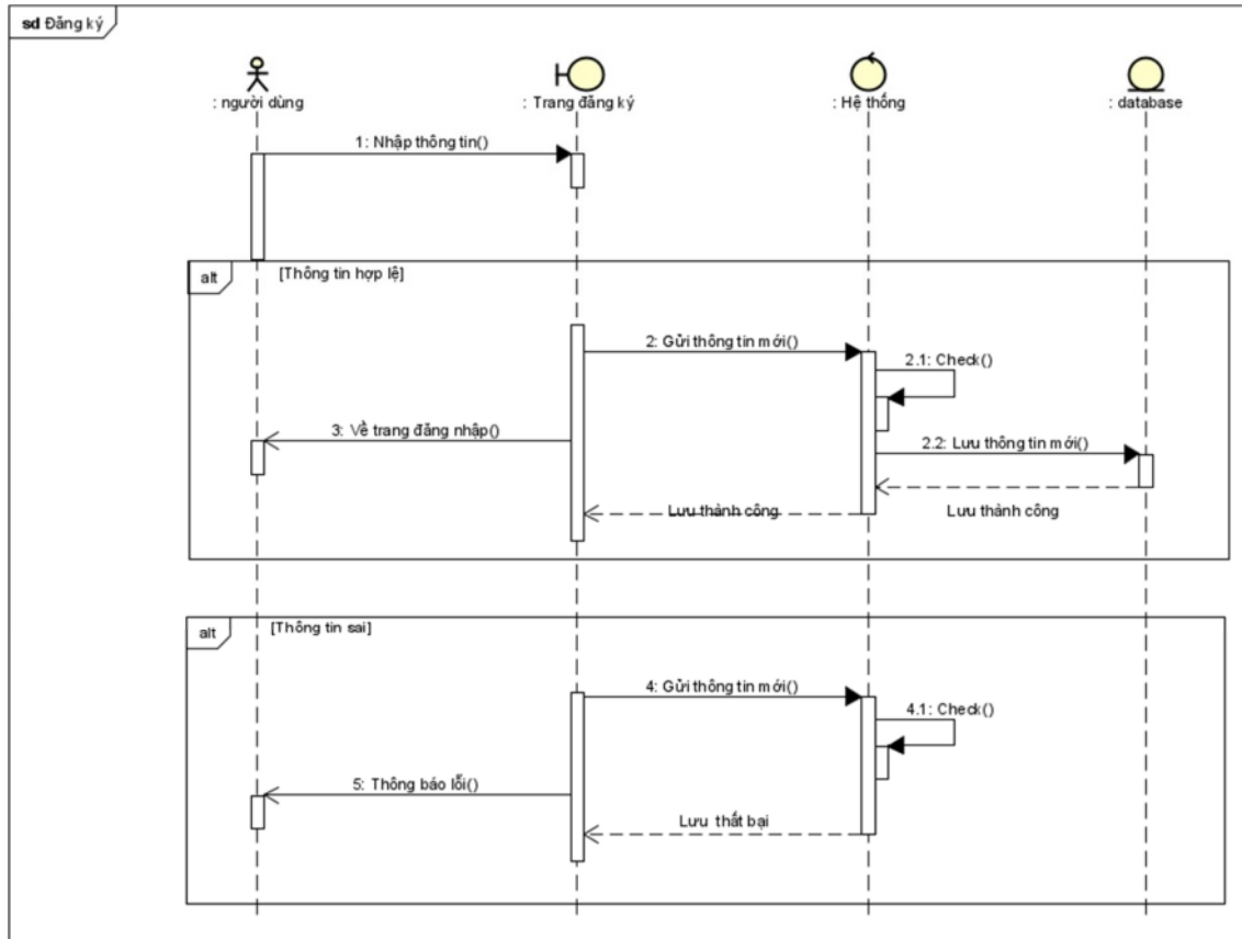
Hình 3.2-17. Hình sơ đồ tuần tự chức năng đăng ký
