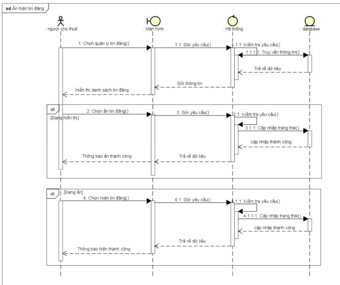
Hình 3.2-25. Hình sơ đồ tuần tự chức năng ấn, hiện tin đăng
