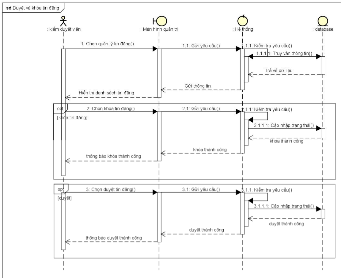
Hình 3.2-26. Hình sơ đồ tuần tự chức năng duyệt, khóa tin đăng
