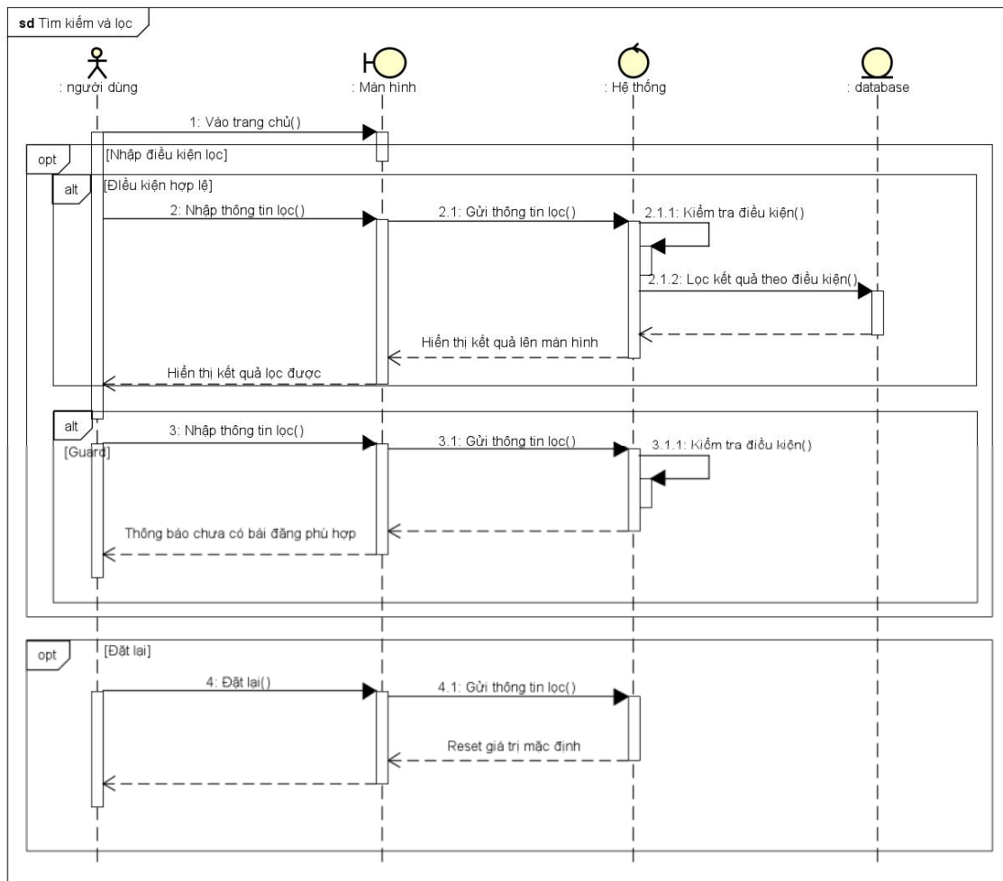
Hình 3.2-19. Hình sơ đồ tuần tự chức năng tìm kiếm và lọc
