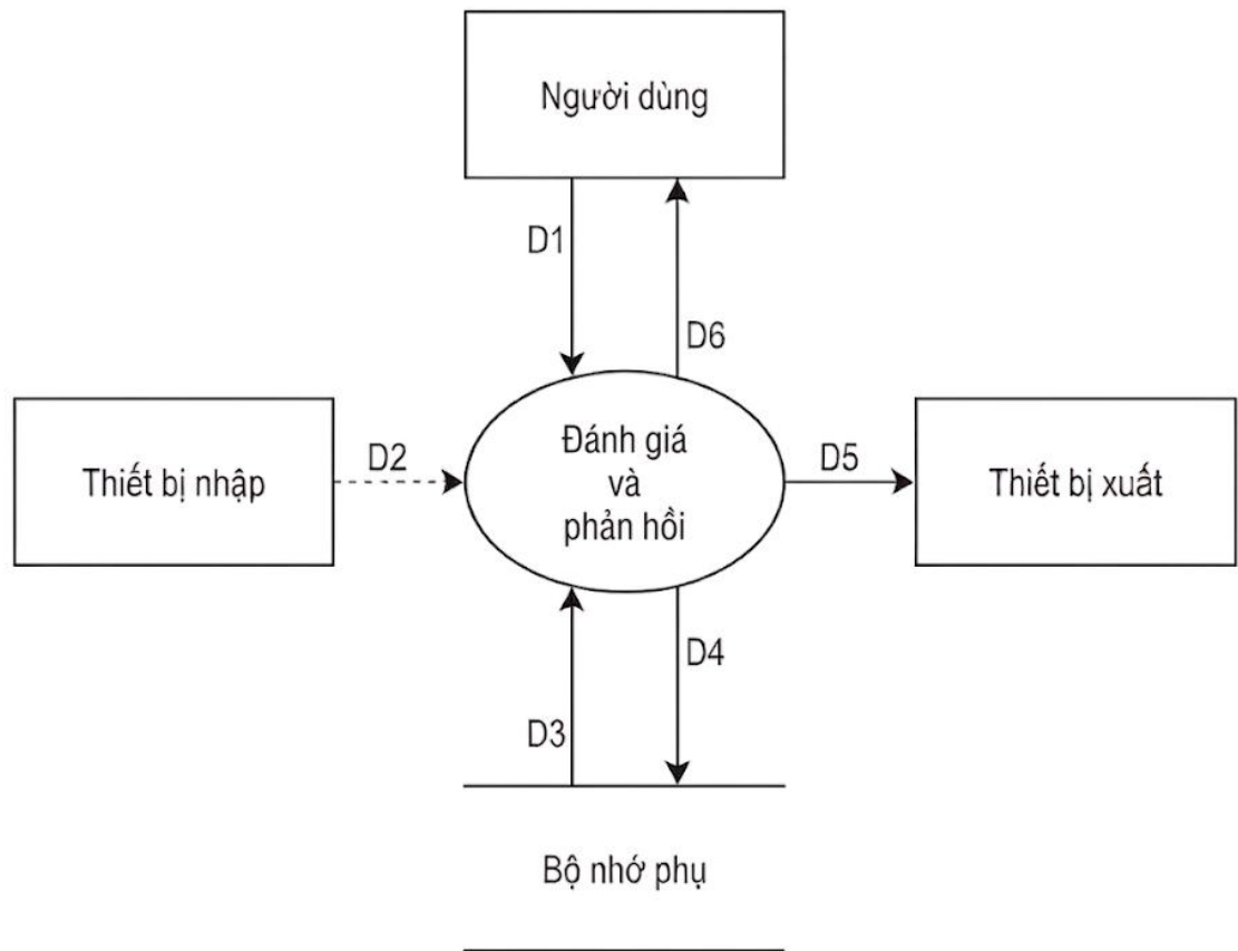
Hình 9. Sơ đồ luồng dữ liệu yêu cầu đánh giá và phản hồi
