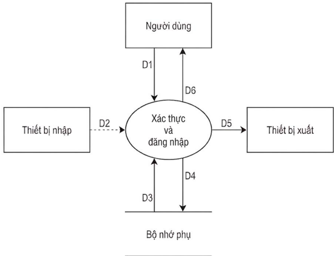
Hình 10.. Sơ đồ luồng dữ liệu yêu cầu đăng nhập
