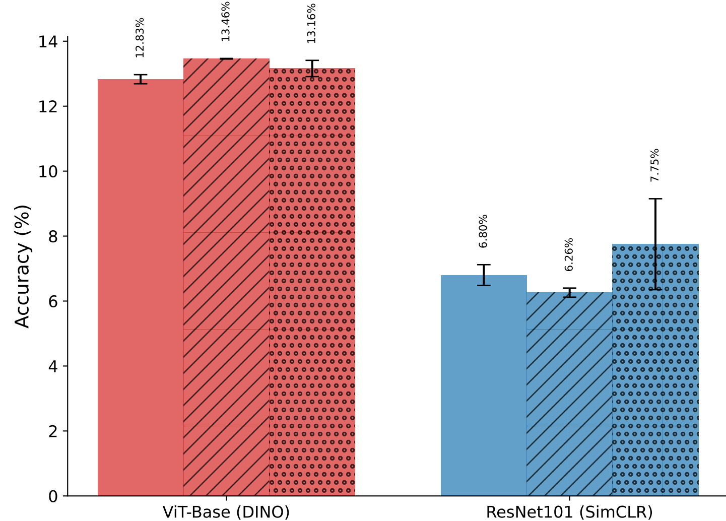
CIFAR100 KNN
