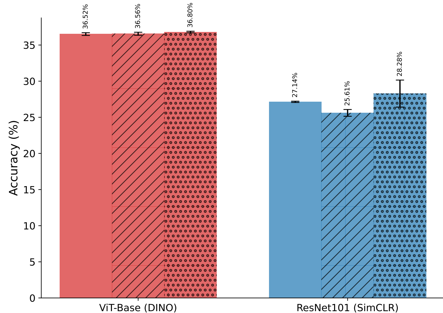
CIFAR10 KNN
