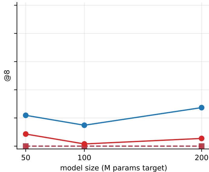
ood
