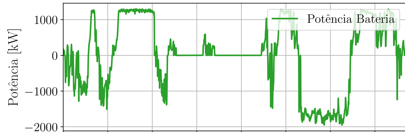
Bateria
