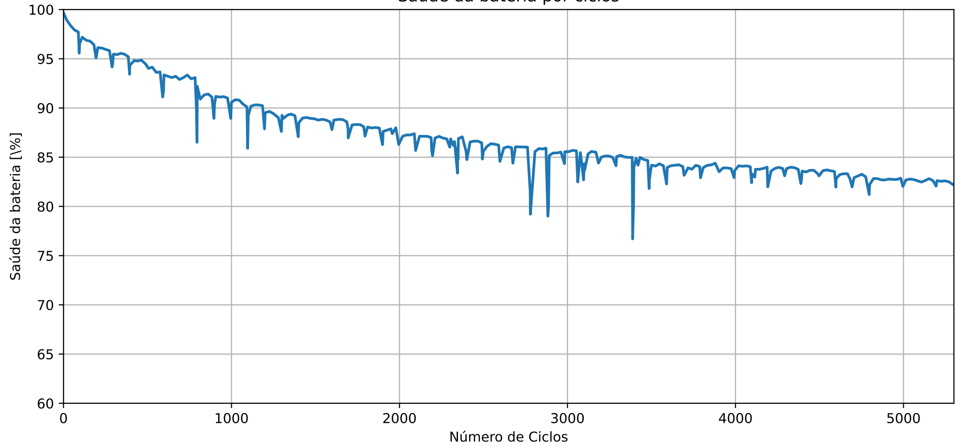
Saúde da bateria por ciclos
