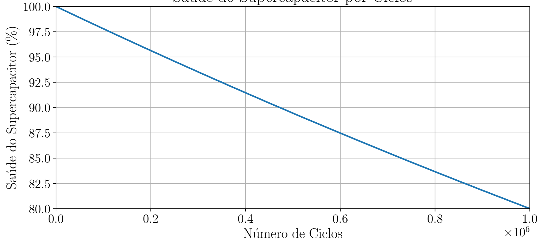
Saúde do Supercapacitor por Ciclos
