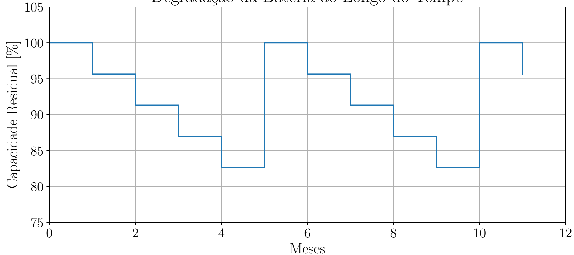
Degradação da Bateria ao Longo do Tempo
