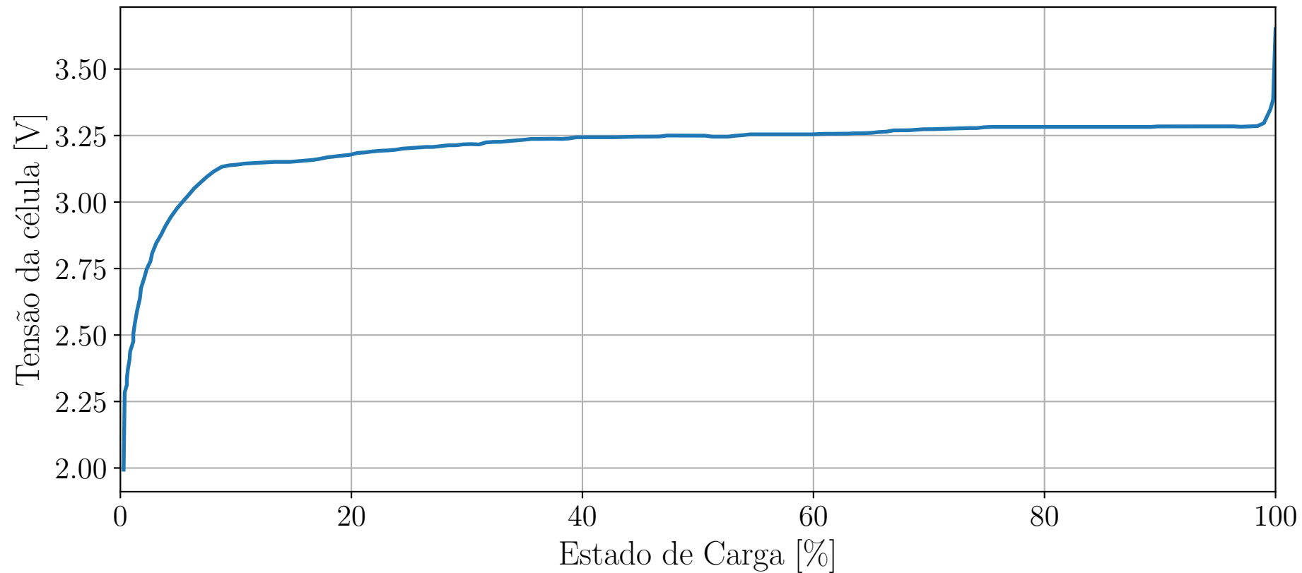
Curva característica da bateria
