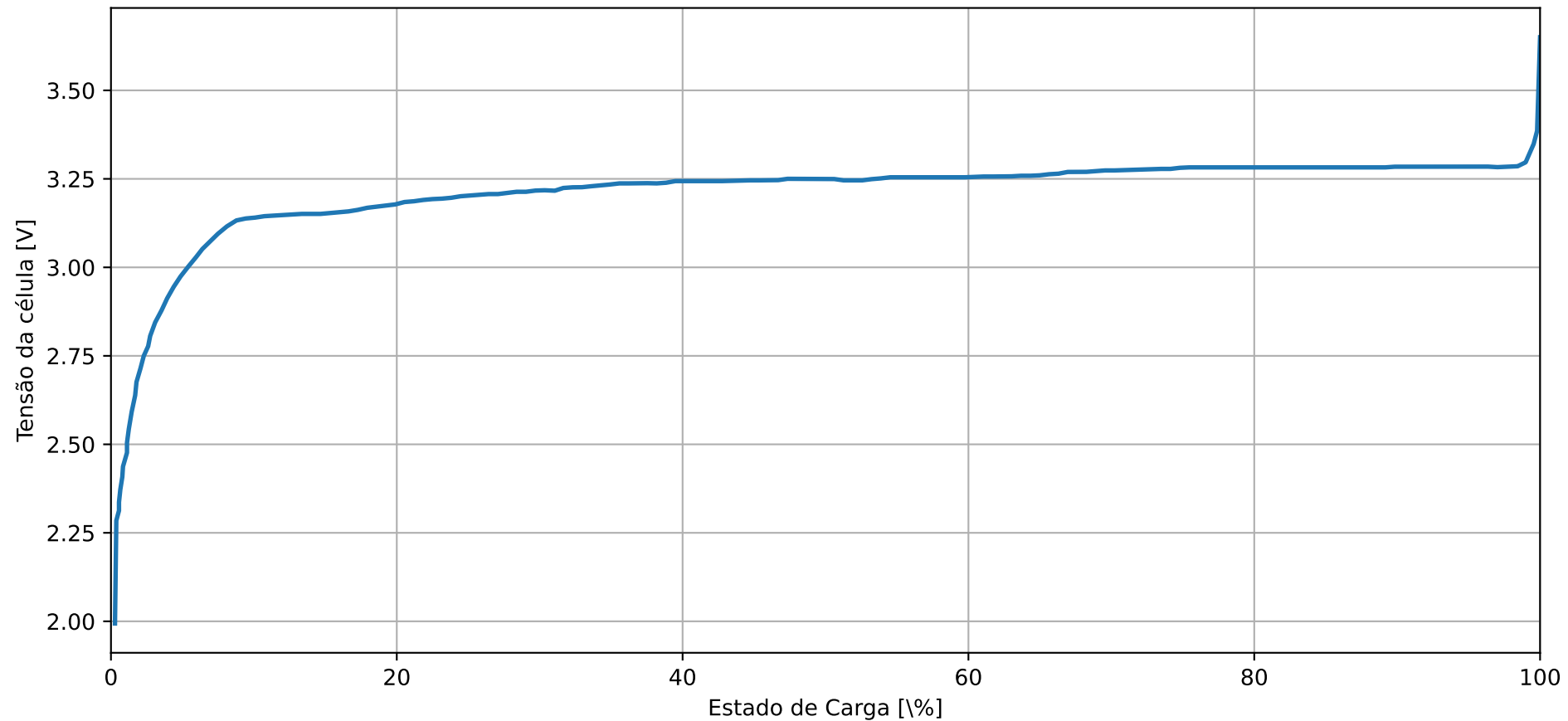
Curva característica da bateria
