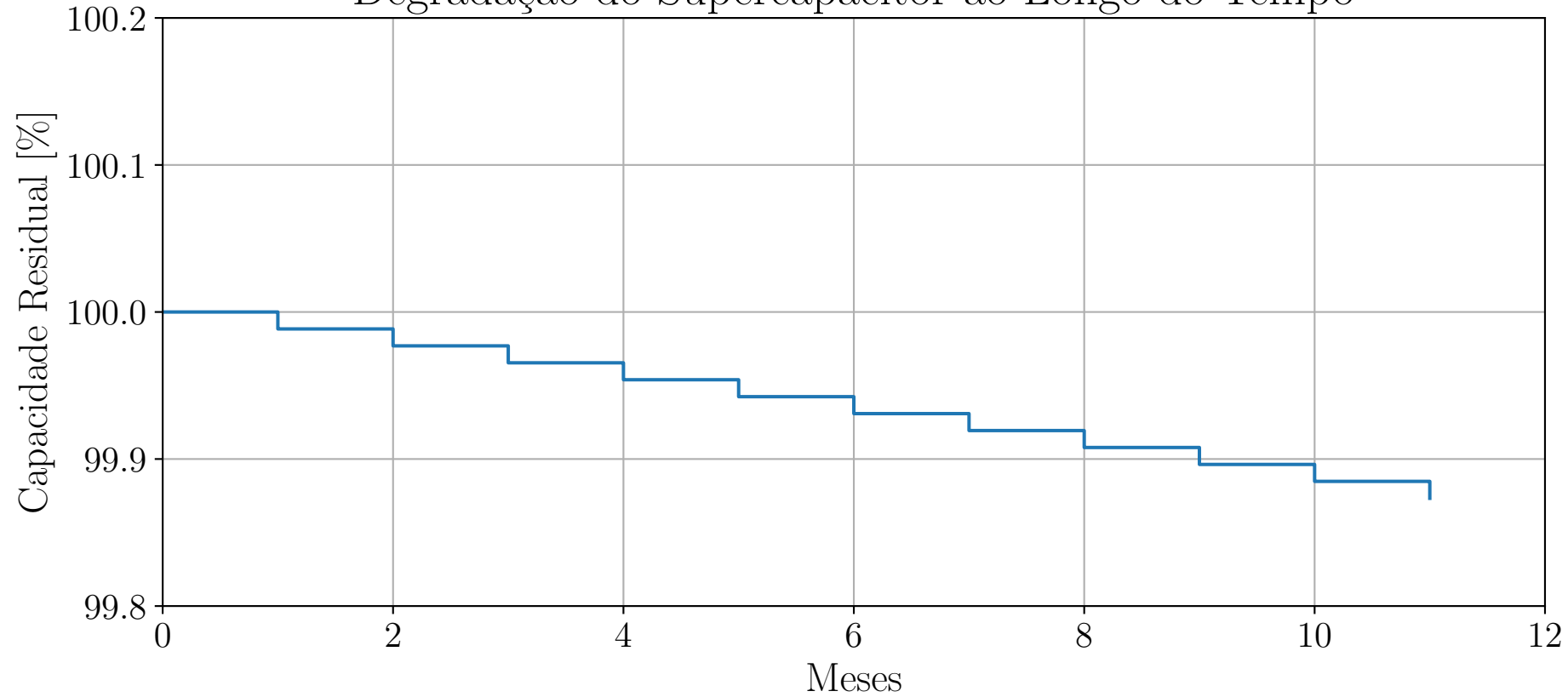
Degradação do Supercapacitor ao Longo do Tempo
