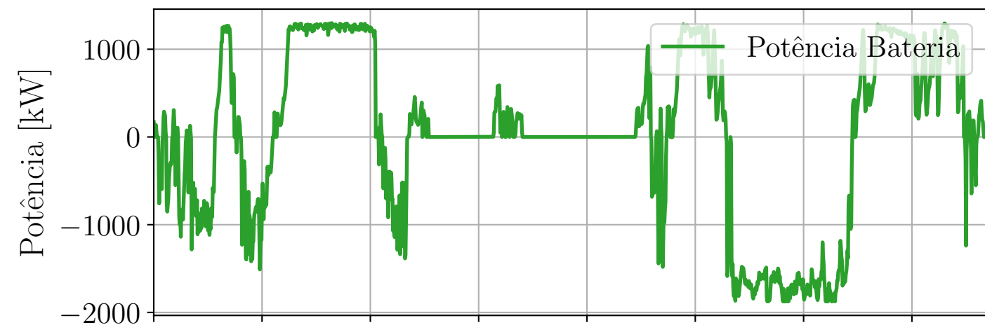
Bateria
