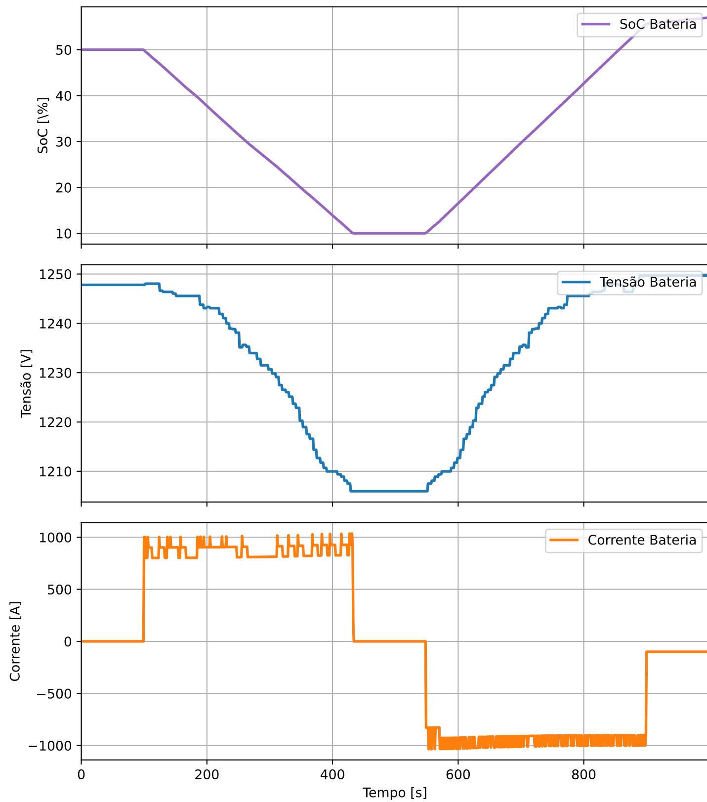
SoC, Tensão e Corrente: Bateria(esq.) x Supercapacitor (dir.)
