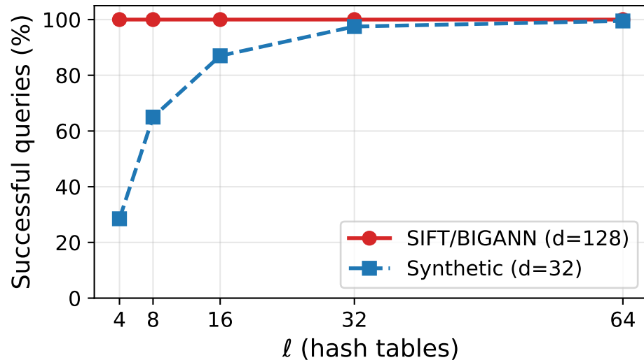
(d) Feasibility vs \ell
